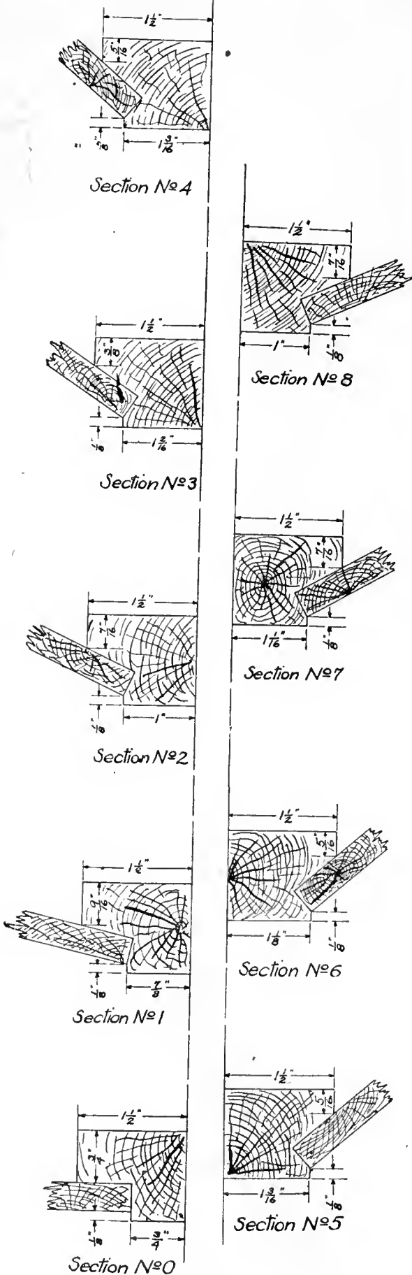
KEEL SECTIONS
