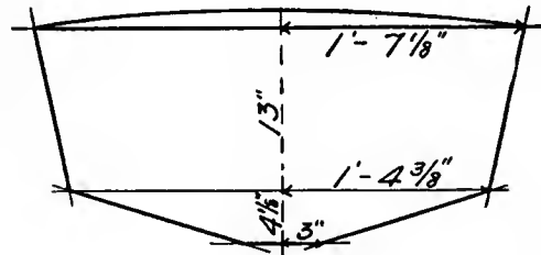
Transom.
