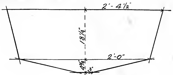
Mould No-2.
