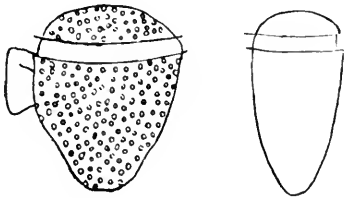
Fig. 21. Phalacroma minutum Cleve in linker Seitenansicht und Dorsal- ansicht. Vergr. 500. Nach Cleve 1900, 3.
