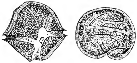
Fig. 88. Peridinium Willei Huitf.-Kaas in Ventralansicht und vorderer Schalenansicht. Vergr. ? Nach Huitfeldt-Kaas.
