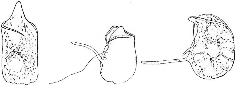
Fig. 135. Gymnodinium pseudonoclituca Pouch.
