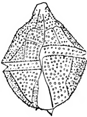
Fig. 36. Gonyaulax polygramma Stein in Ventralansicht. Vergr. 440. Nach Paulsen 1907.
