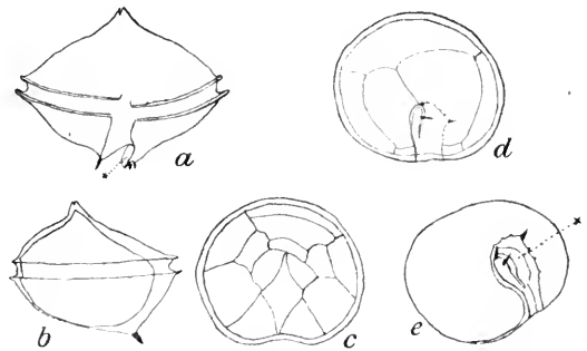
Fig. 62. Peridinium islandicum Pauls. a: ventrale Gürtelansicht, b: rechte Seitenansicht, d, e: antapicale, c: apicale Gürtelansicht. x: Flügelstachel.
