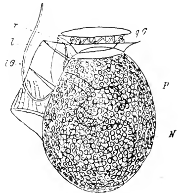
Fig. 16. Dinophysis ovum Schütt in linker Seitenansicht. P : Pusule. N : Kern. qG : Quergeißel. r : Rechte Längsfurchenleiste. l : Linke Längsfurchenleiste. IG : Längsgeißel. Vergr. 640. Nach Schütt 1895.
