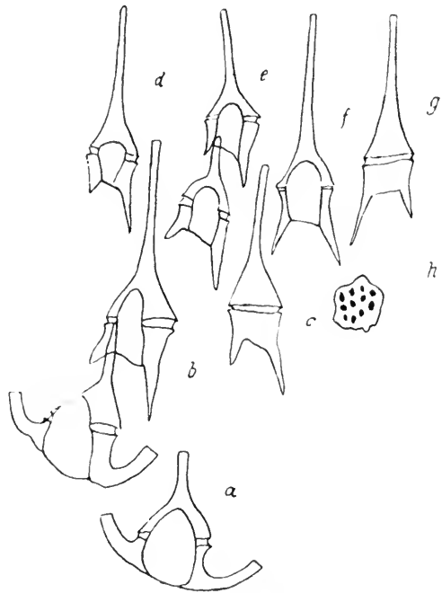
Fig. 106. a: Ceratium tripos f. truncata Lohm. b: Kette von f. lineata und f. truncata . c—g: f. lineata . h: Panzerstruktur. Nach Lohmann 1908.
