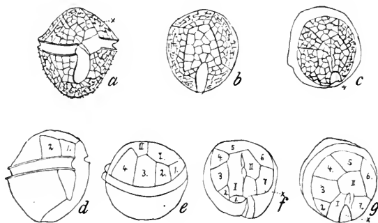
Fig. 33. Protoceratium reticulatum (Clap. u. Lachm.) Bütschli.
