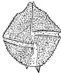
Fig. 37. Gonyaulax spinifera (Clap. u. Lachm.) Dies. in Ventralansicht. Vergr. ca. 420. Nach Paulsen 1907.
