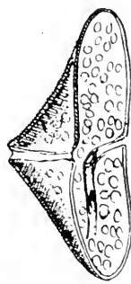
Fig. 25. Glenodinium foliaceum Stein in Dorsalansicht und rechter Seitenansicht. Vergr. ? Nach Stein.
