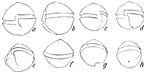
Fig. 27. Glenodinium danicum Pauls. a—b : Ein Exemplar, c—h : ein anderes. a, c, d, e : Verschiedene Ventralansichten. b, h : Linke und rechte Seitenansicht. f, g : Dorsalansichten. Vergr. 460. Nach Paulsen 1907.
