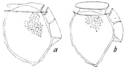
Fig. 12. Dinophysis norvegica Clap. u. Lachm. a : var. crassior , von der Murmañküste. b : var. debilior , von der Ostsee. Vergr. 460. Nach Paulsen 1907. (Skulpturierung nur angedeutet.)
