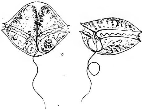
Fig. 30. Glenodinium obliquum Pouchet in Ventralansicht und etwas von der linken Seite. Das Exemplar links zeigt Teilung im beweglichen Zustand. o : Öffleck. Vergr. ca. 400. Nach Klebs 1884.
