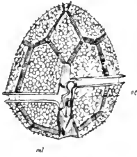
Fig. 87. Peridinium tabulatum Ehbg. ml : Geschlängelte Leiste. oc : Stigma. Vergr. ? Nach Stein.
