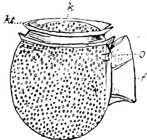
Fig. 18. Dinophysis rotundata Clap. u. Lachm. in rechter Seitenansicht. kt. : Vorderkörper. kt. : Kopftrichter. f. : „Henkel“. o. : Geißelspalt. Vergr. ? Nach Stein.
