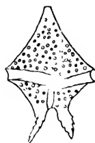
Fig. 152. Peridinium exiguum Cleve in ventraler Gürtelansicht. Vergr. 500. Nach Cleve 1900, 3.
