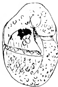
Fig. 147. Pouchetia nigra (Pouch.) Lemm. Schwarzer Pigmentkörper geplatzt. Vergr. 500. Nach Pouchet 1887.
