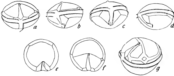
Fig. 45. Diplopsalis lenticula Bergh. f. minor Paulsen. a, b, c : Ventralansicht, d, g : Linke Seitenansicht. e : Antapicale, f : Apicale Schalenansicht (beide etwas schematisiert). a—d : Dasselbe Exemplar. In a zeigt sich die breite Flügel- leiste des Längsfurchenrandes unten wie ein Dorn. Vergr. 460. Nach Paulsen 1907.
