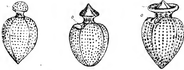
Fig. 90. Oxytoxum sphaeroideum Stein.
