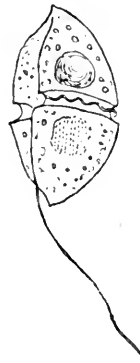
Fig. 26. Glenodinium Gymnodinium Pénard in linker Seitenansicht und Ven- tralansicht. Vergr. 625. Nach Pénard.
