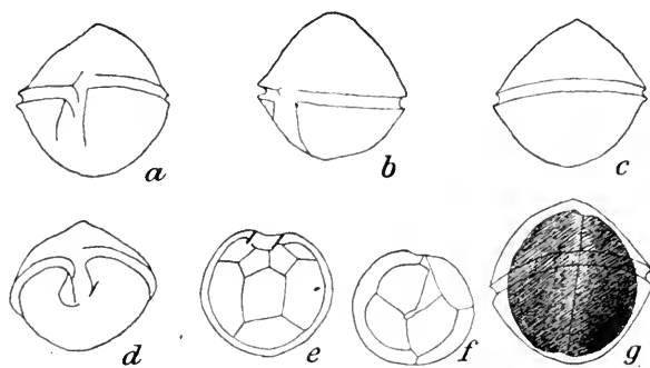
Fig. 43. Goniodoma Ostenfeldii Pauls. a, b, d: ventrale, c, g: dorsale Gürtelansicht, in g hat sich der Inhalt geteilt. e: antapicale, f: apicale Schalenansicht. Vergr. ca. 350.
