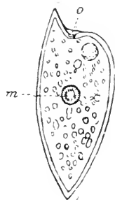
Fig. 3. Procoenocentrum dentatum Stein
