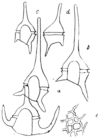
Fig. 105. a: Kette von Ceratium tripos und f. lata Lohm. b—d: f. lata . e: Panzerstruktur. Nach Lohmann 1908.
