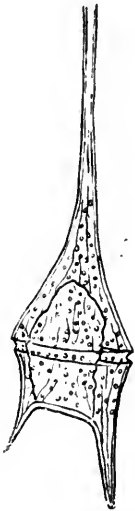
Fig. 121. Ceratium tripos f. lineatum (Ehbg.) Lohm. in ventraler Gürtelsicht. Vergr. ? Nach Bergh 1881.
