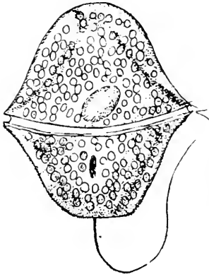
Fig. 25. Glenodinium foliaceum Stein in Dorsalansicht und rechter Seitenansicht. Vergr. ? Nach Stein.
