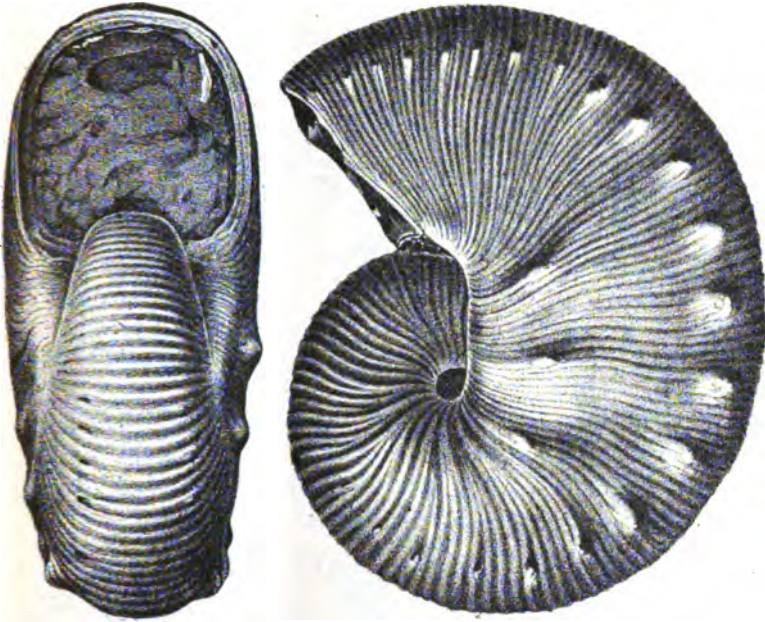
FIG. 1428. Scaphites nodosus var. brevis . (Alter Meek.)
