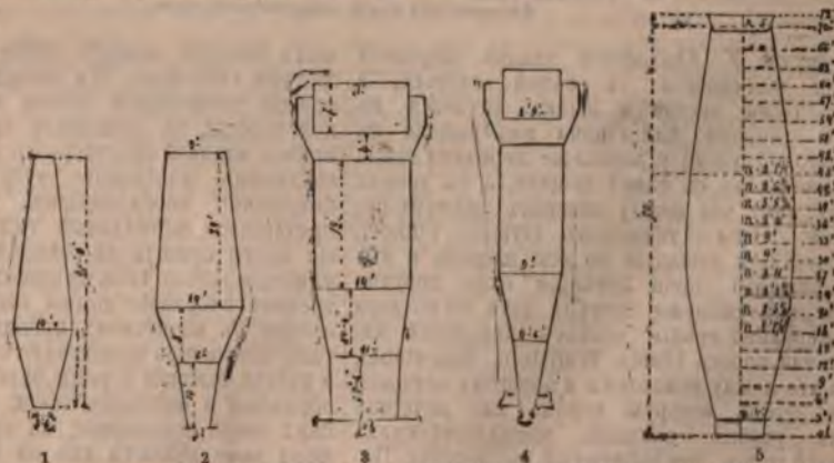
1) Вертикальный разрѣзъ 1) блюофена 2) доменъ для древесно-угольного топлива, 3 и 4) доменной печи Рашета и 5) коксовой доменъ.
