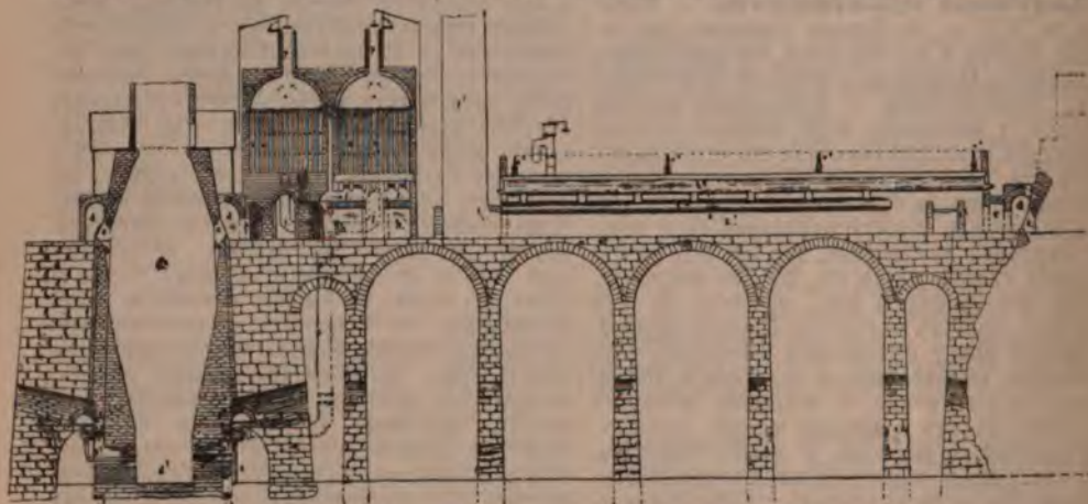
Антрацитова домна американскаго типа.
