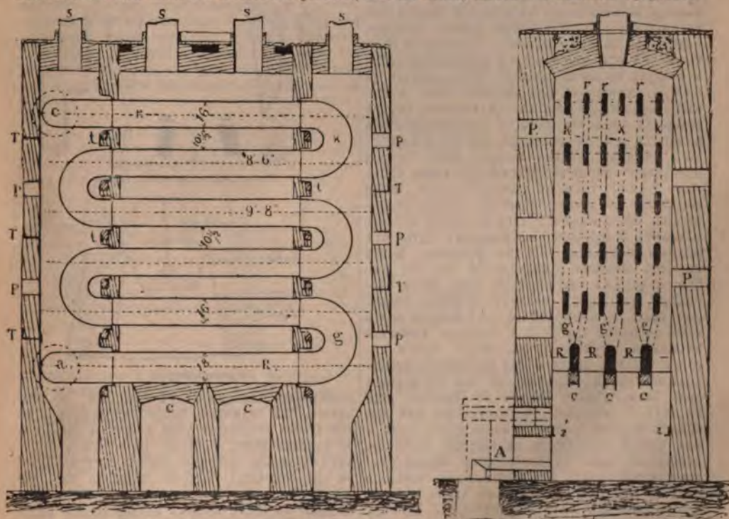
Вассер-альфингенскій воздушнонагрѣвательный аппаратъ.
