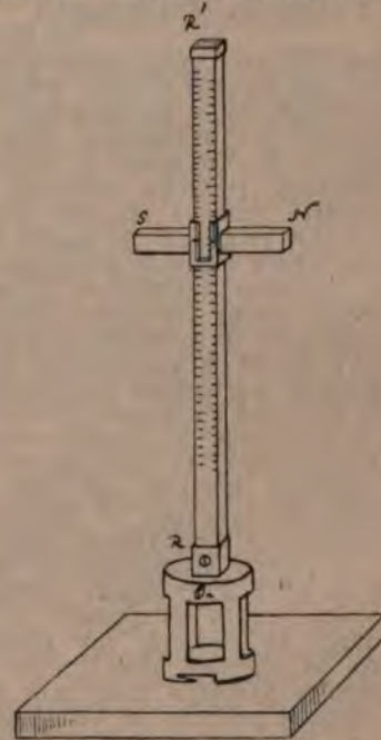
Дефлекторъ (внизу въ открытую коробку вставляется магнитикъ, направленный перпендикулярно большому магниту NS ).
