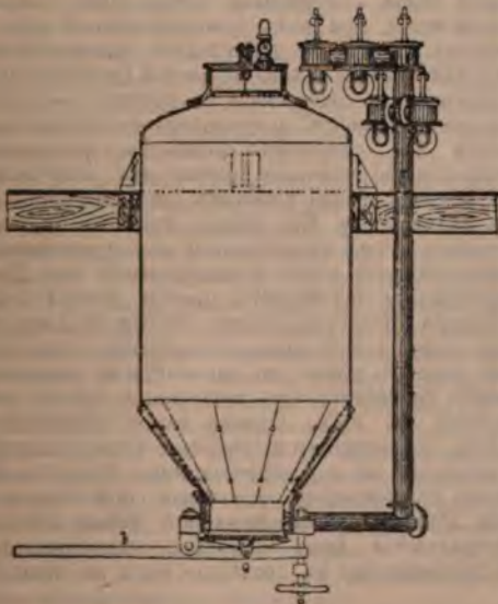
Фиг. 2. Одинъ диффузоръ для извлеченія сока изъ са- харовицы рѣзки.
