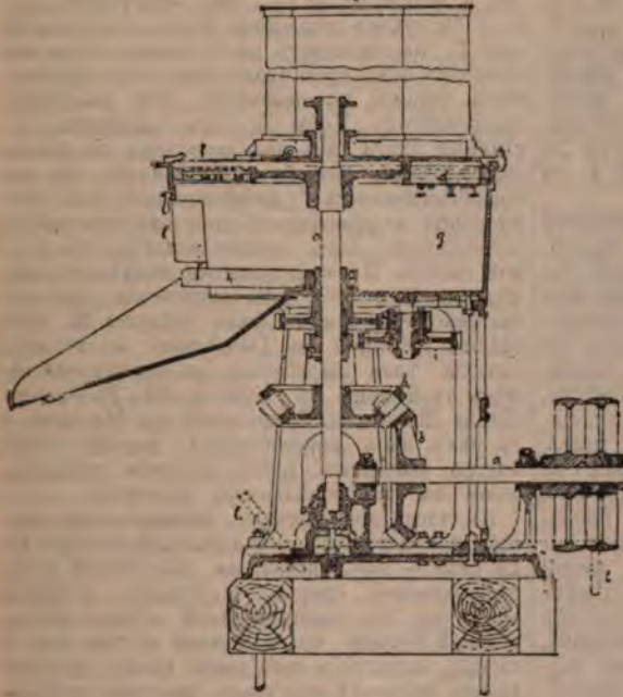
Фиг. 1. Рѣзка сахаровицы для диффузіи.
