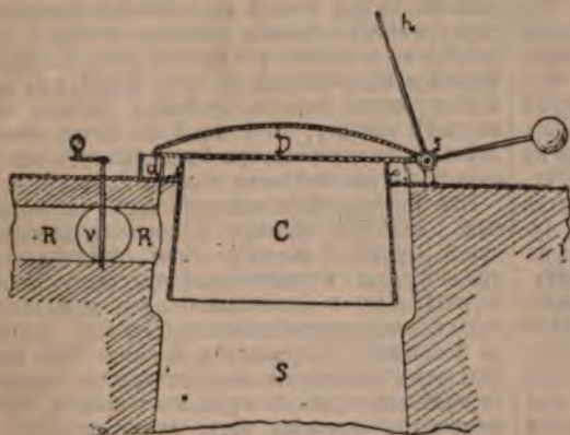
Способъ улавливанія колошниковыхъ газовъ.
