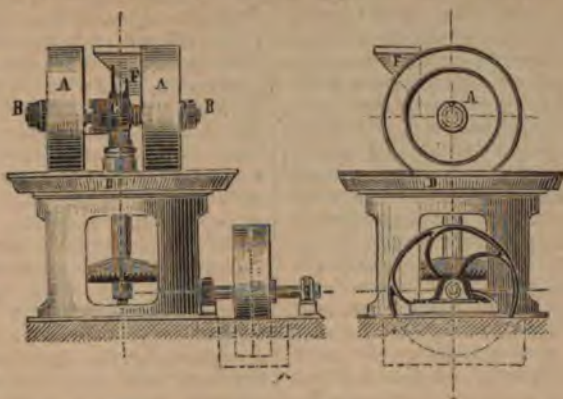
Бѣгунъ, общій видъ.
