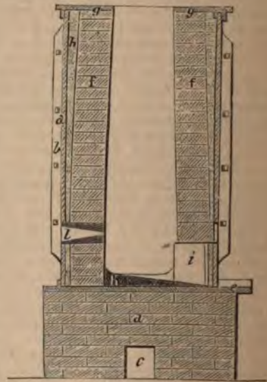
Вагранка, вертикальный разрѣзъ.
