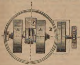
Бѣгунъ, видъ сверху.
