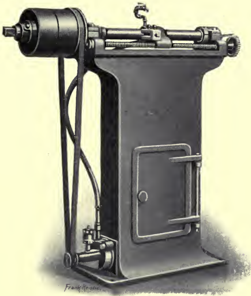
FIG. 80. ZINC LATHE.
