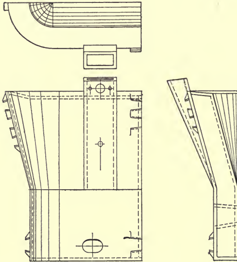
FIG. 138. CAST-IRON END-JACKET.
