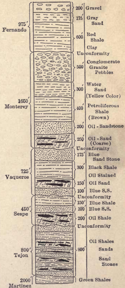
FIG. 7.—Geologic column.
