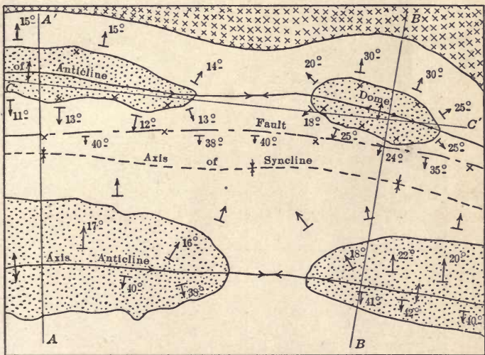
FIG. 31.—Geologic map.
