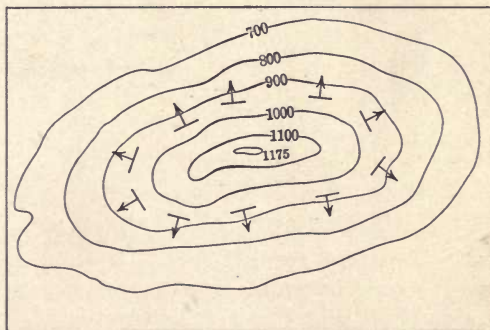
FIG. 28.—Dome.
