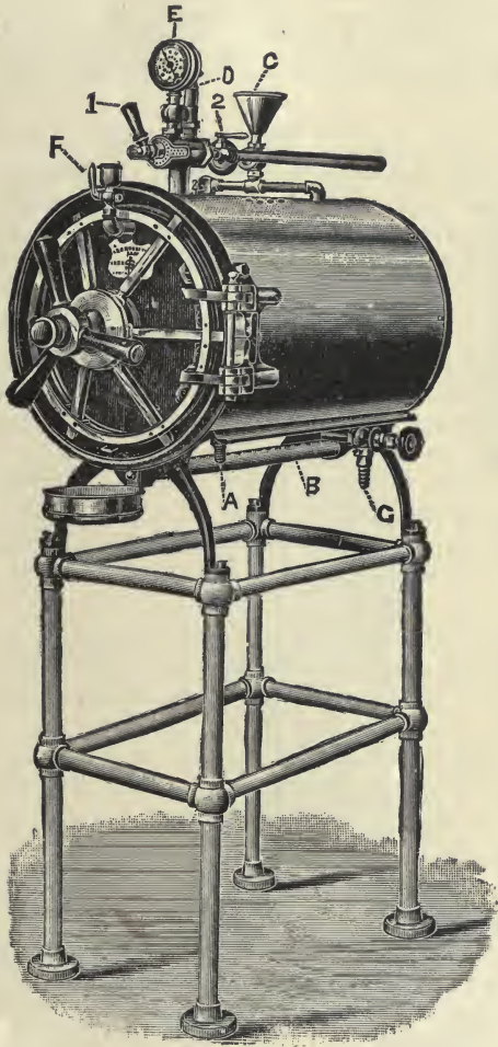
FIG. 4.—AUTOCLAVE.
