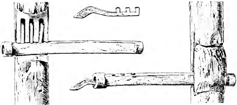
Abb. 5. Türverschluß bei den Makonde, aus Wenke, Negerleben in Ostafrika. Leipzig, Brockhaus 1909.
