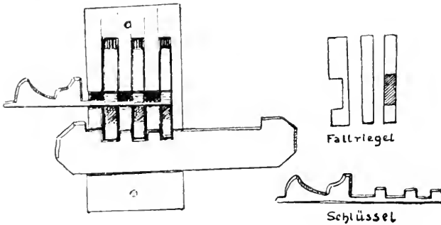
Abb. 6. Türschloß aus einem Araberhaus in Sansibar, nach Stuhlmann
