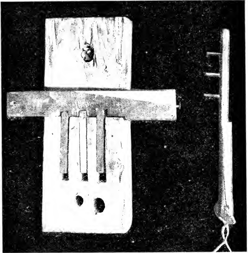
Abb. 8. Schloß und Schlüssel einer Waldmühle in der Biegerschlucht bei Millstatt Kärnten; Ende des 18. oder Anf. des 19. Jahrh. Jetzt dort durch ein genaues Facsimile ersetzt. Etwa \frac{1}{4} der natürlichen Größe.
