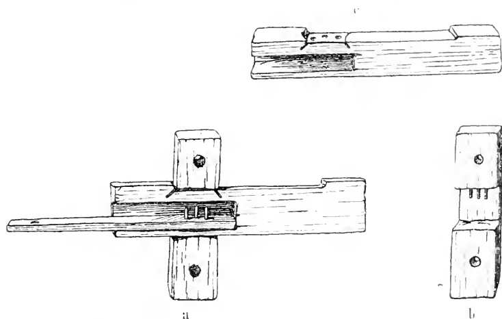
Abb. 7. Türschloß aus Assuan. Etwa \frac{1}{2} der natürlichen Größe; a) Das vollständige Schloß, b) Der Schloßkasten mit den herabgefallenen drei eisernen Stiften, c) Der Querriegel. Mit gütiger Erlaubnis von L. Friederichsen & Co. reproduziert aus Meinhof, Studienfahrt nach Kordofan. Hamburg 1916.
