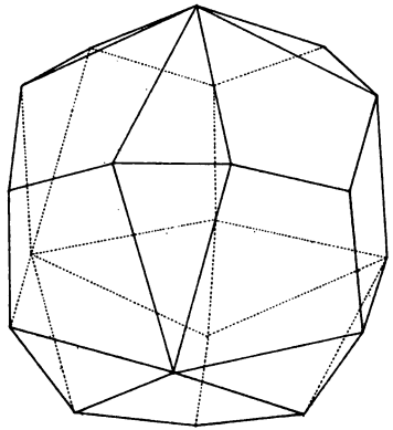
Penta-Tetraeder.
