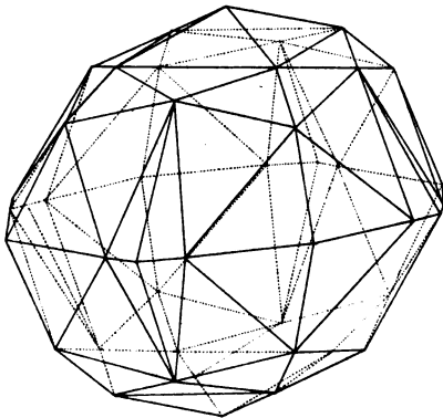
Octocontaeder.
