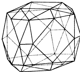
12. Würfel-Hexa-Tetraeder.
