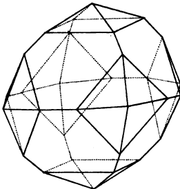
11. Pyramiden-Hexa-Tetraeder.
