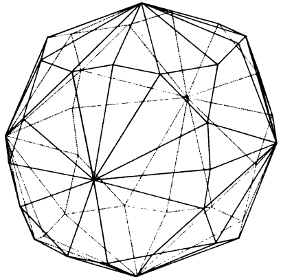
25. Hepta-Octaeder.
