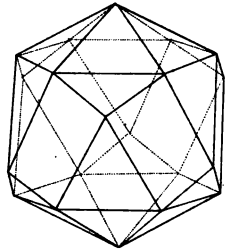
10. Hexa-Tetraeder.
