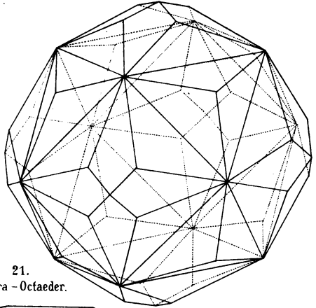
20. Pyramiden-Trioctaeder.
