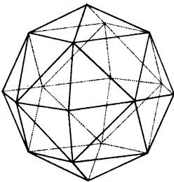
11. Pyramiden-Hexa-Tetraeder.
