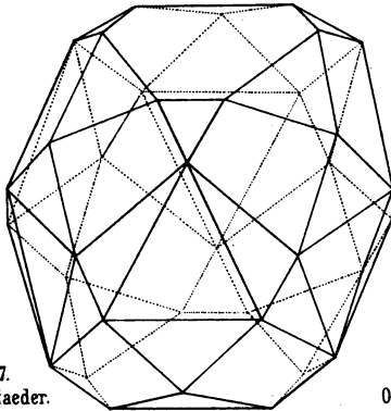
Octocontaeder.
