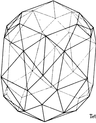
19. 1. Heptacontaeder.
