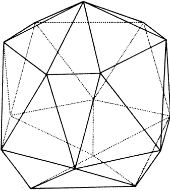
Tetra-Tetraeder.
