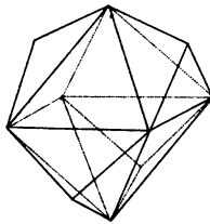
9. Trapezoeder.
