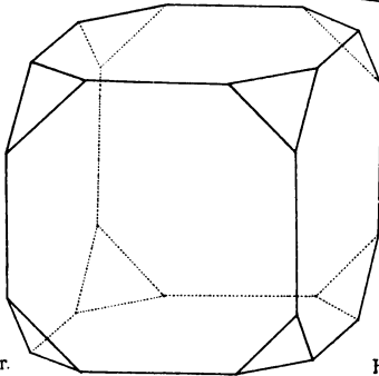
21. Tetra-Octaeder.
