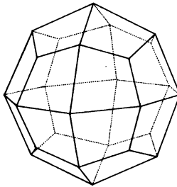
12. Würfel-Hexa-Tetraeder.
