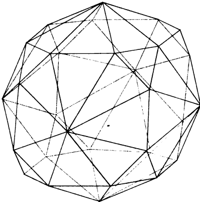
22. Penta-Octaeder.
