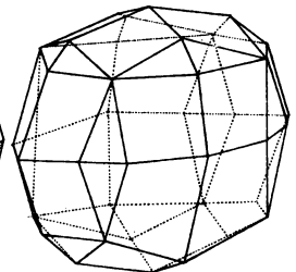
13. Amphieder.
