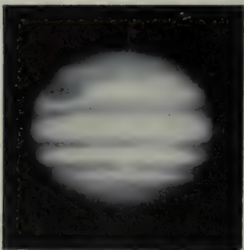
FIG. 12.—JUPITER
