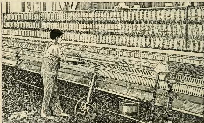
FIG. 92. SPINNING MULE
