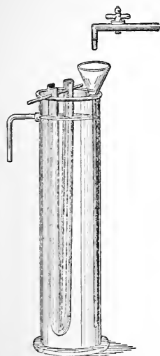
Fig. 10. Kühne's Dialyser.
