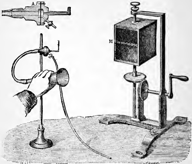
Fig. 119. —Koenig's Manometric Flame Apparatus.
