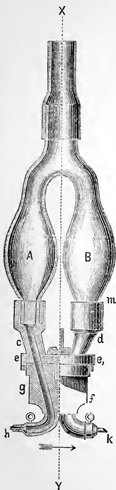
Fig. 111—Rheometer.
