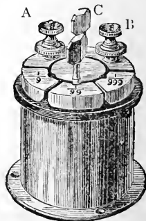
Fig. 81.—The Shunt.
