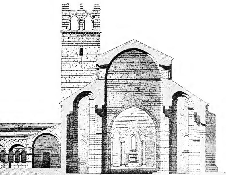
FIG. 100. — Cathédrale de Vaison.
