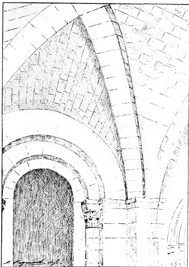
FIG. 208. — Porche de Saint-Victor de Marseille.
