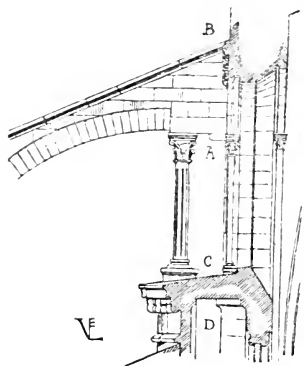
FIG. 251. — Arc-boutant de Saint-Remi de Reims. ( Annales archéol. )
