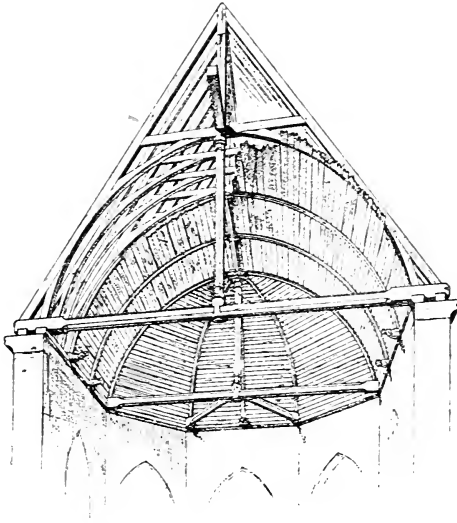
FIG. 240. — Lambris de Tillard (Oise).
