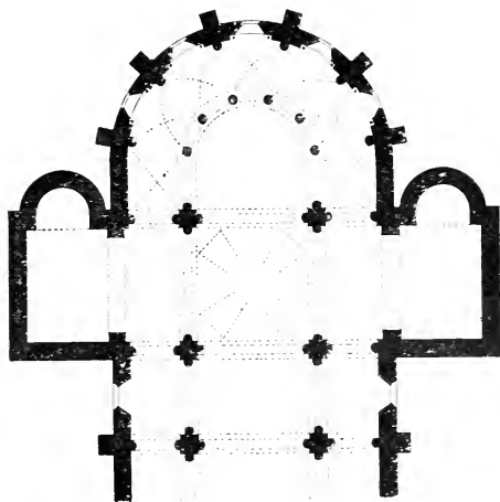
Fig. 76. — Chœur et transept de Saint-Saturnin Puy-de-Dôme.
