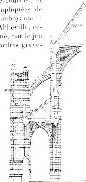
FIG. 327. — Coupe de Saint-Martin d'Argentan Orne. Archives de la Commission des Monuments historiques.
