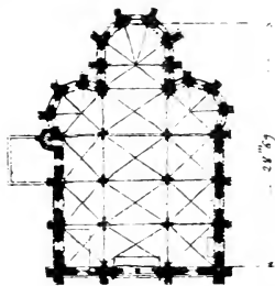
FIG. 232. — Église de Villeneuve-le-Comte (Seine-et-Marne). Archives de la Commission des Monuments historiques).
