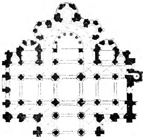
Fig. 82. — Chœur et transept de Conques (Aveyron).
