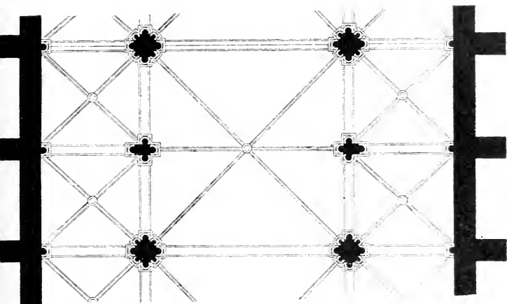
Fig. 223. — Voûte sexpartite du XIII e siècle à Pont-sur-Yonne. Ann. archéol.
