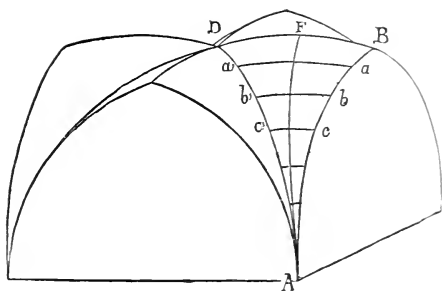
Fig. 15. — Tracé d'une voûte d'arêtes brisée. Ann. Archéol.
