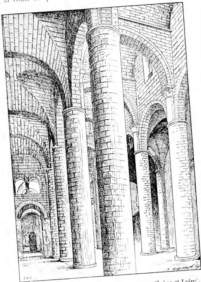
FIG. 103. — Nef de Saint-Philibert de Tournus (Saône-et-Loire).
