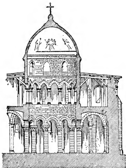
FIG. 65. — Église de Neuvy-Saint-Sépulchre.
