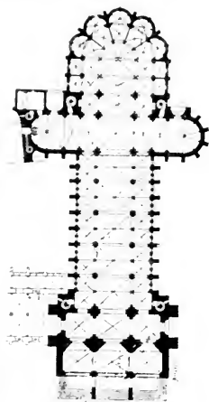
Fig. 228. Cathédrale de Noyon.
