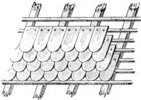
FIG. 28. — Chevrons, pannes, tuiles, ardoises ou essauls imbriqués. (Mél. Quicherat, t. II.)
