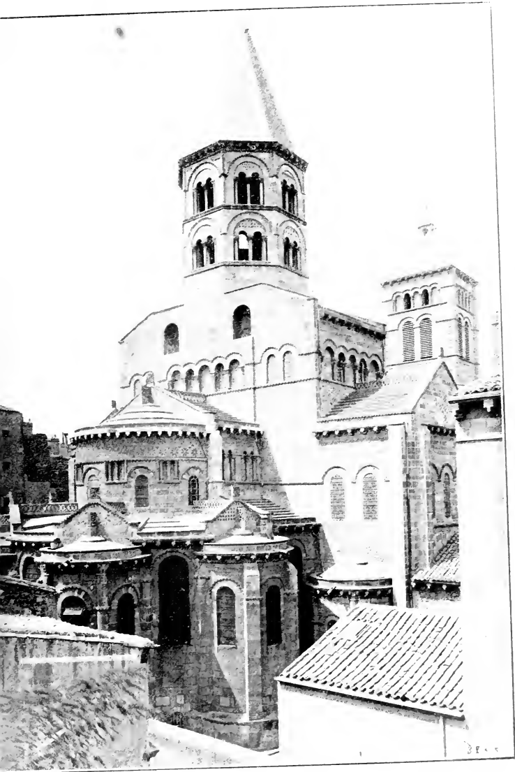
Fig. 140 — Abside et clocher central de Notre-Dame-du-Port à Clermont. (Phot. de la Commission des Monuments historiques.)
