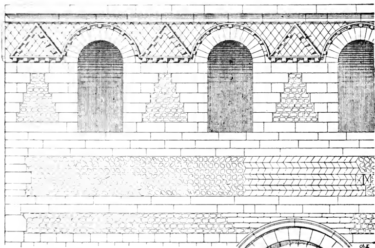
Fig. 1. — Église carolingienne de Cravant (Indre-et-Loire).
