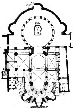
FIG. 64. — Église du Saint-Sépulchre, à Jérusalem.
