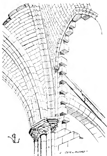
Fig. 16. — Voûtes d'ogives. Ann. Archéol.
