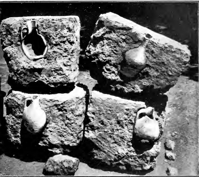
FIG. 350. — Vases acoustiques de l'église des Carmes de Famagouste vers 1360.
