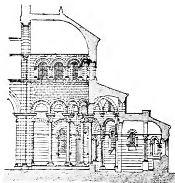
FIG. 83. — Abside de Paray-le-Monial Mél. Quicherat, t. II.
