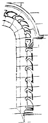
Fig. 153. — Fenêtre de façade, Coudun (Oise).
