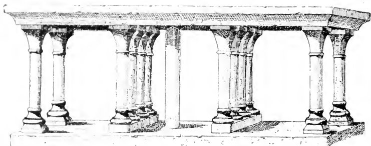
FIG. 367 bis. — Maître-autel de Poblel (Catalogne, seconde moitié du XII e s.)
