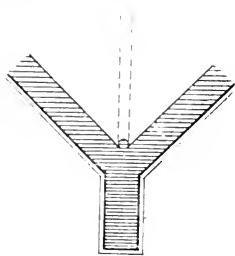
FIG. 258. — Contrefort normal à un angle.
