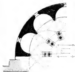
FIG. 79. Abside de la cathédrale de Trier.
