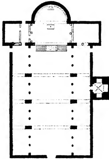
FIG. 44. — Sainte-Praxède à Rome.
