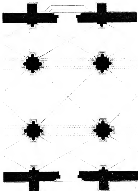
FIG. 109. — Nef de Pont-Aubert (Yonne . Annales archéol. ).
