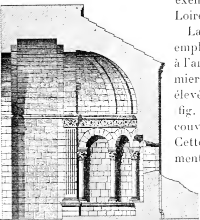
FIG. 114. — Abside de Saint-Jean-du-Moutier à Arles. Revoil. Archit. romane du Midi .
