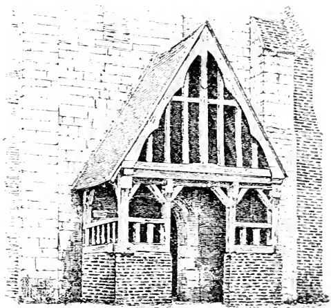
FIG. 319. Porche de Mareuil-Caubert Somme 1 .
