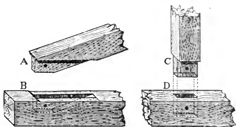
Fig. 25. — Tenons et mortaises. Mél. Quicherat, t. II.
