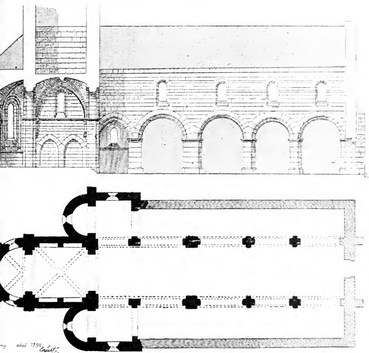
FIG. 215. — Plan et coupe de l'église de Quesmy (Oise). Transition: milieu du xii e siècle.
