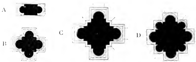
FIG. 132. — Piliers composés à colonnes engagées.
