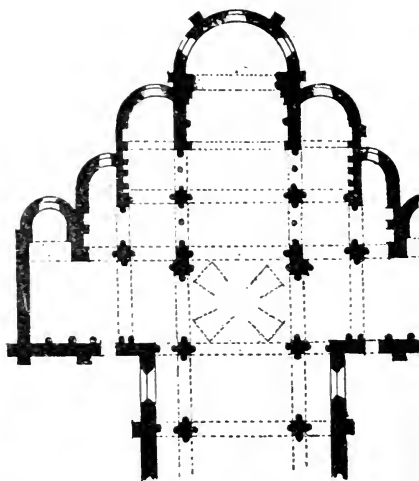
FIG. 75. — Chœur et transept de Château (Cher).
