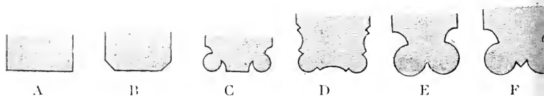
FIG. 218. — Évolution du profil à épannelage carré.
