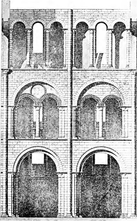
FIG. 97. — Nef de Cerisy-la-Forêt (Manche). (Rüprich-Robert, Arch. normande .)
