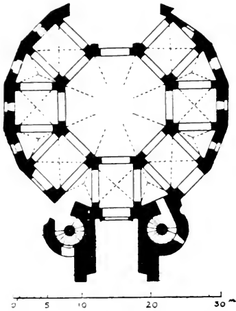
FIG. 47. — Chapelle palatine d'Aix.
