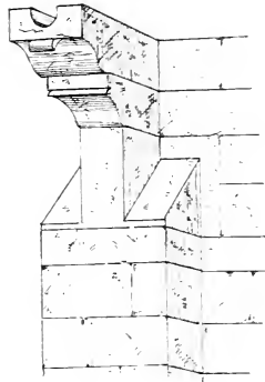
Fig. 200. Gargouille à Fontenay Côte-d'Or.
