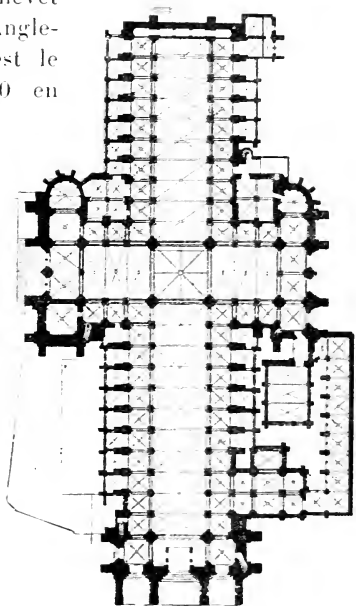
FIG. 231. — Cathédrale de Laon.
