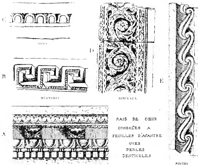
FIG. 147. — Ornaments romans d'origine classique.
