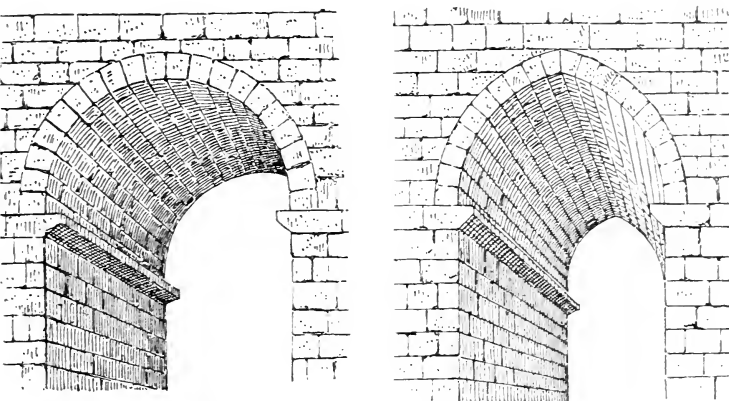
Fig. 13. — Voûtes en berceau.
