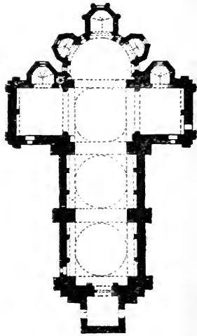
FIG. 77.— Souillac II e -Vienne
