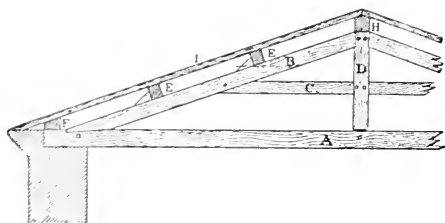
Fig. 26. — Ferme. Mét. Quicherat , t. II.
