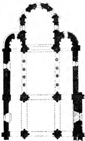
FIG. 74. — Chœur et transept de Saint-Genou (Indre).
