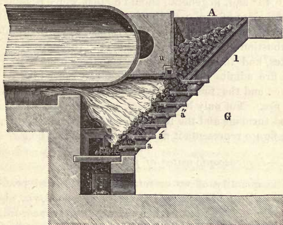
Fig. 1.—STAIR GRATE.
