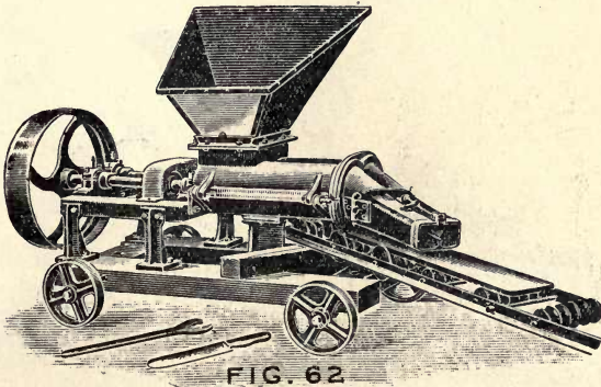
FIG. 62—R. Dolberg's Peat Machine No. 1a (exterior).
