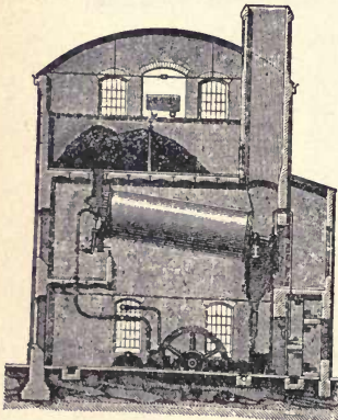
Schulz Drier.
