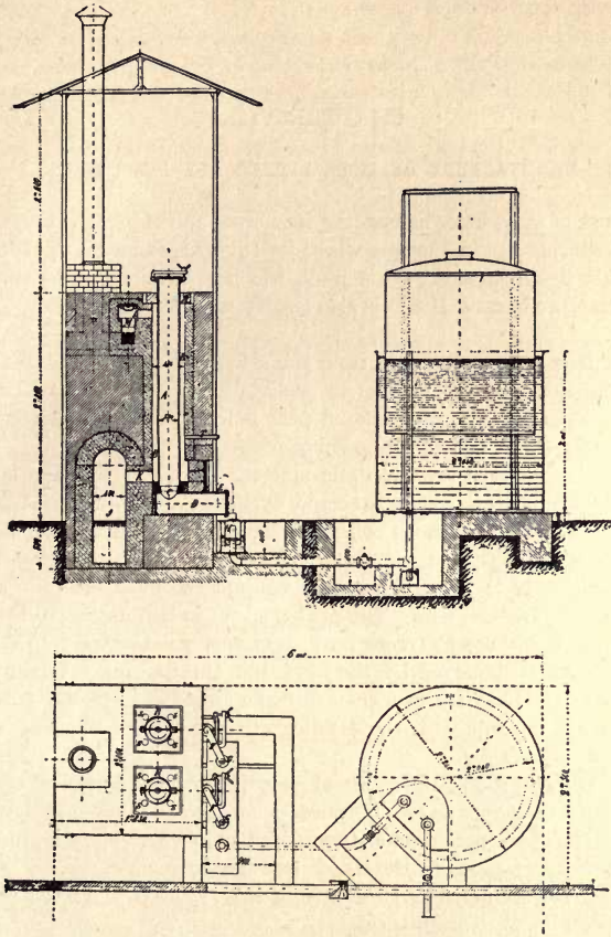
FIG. 212—Riché Gas Plant.
