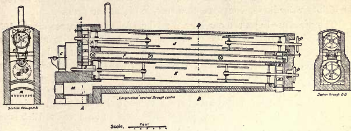
FIG. 164—The Simpson Drier.
