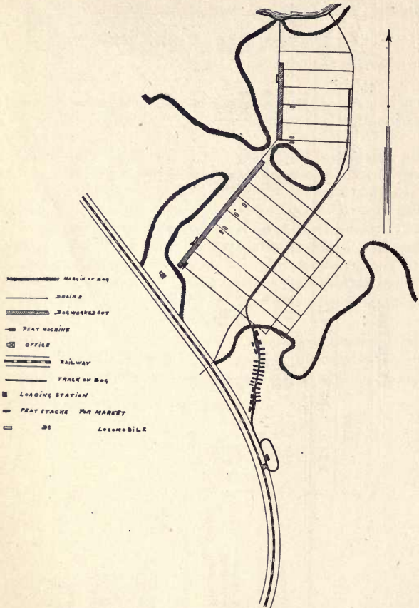
FIG. 128—Peat Bog at Koskivara, Sweden.
