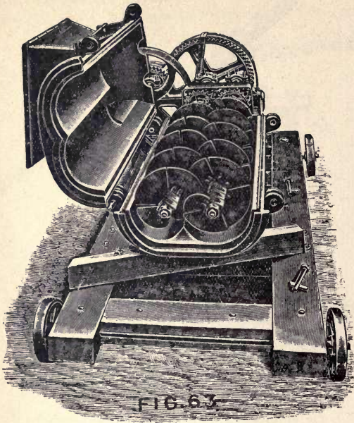
FIG. 63—R. Dolberg's Peat Machine No. 1a (interior).
