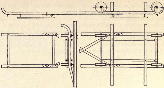
FIG. 111—Carrier.
