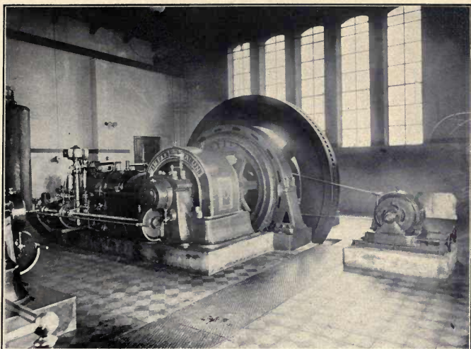
Gas Engine at Skabersjö Peat-gas Plant, Sweden.
