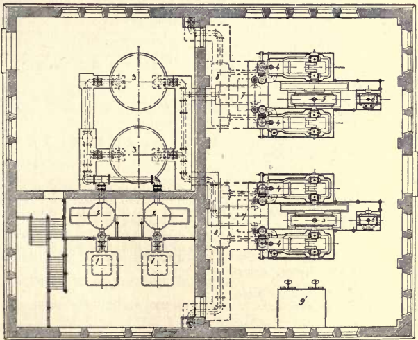
Peat-gas Power Plant at Skabersjö, Sweden.
