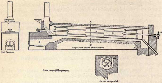
FIG. 168—The Dobson Drier.
