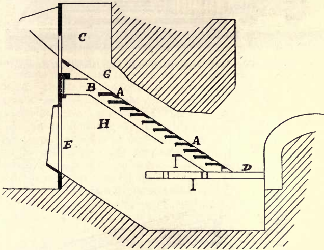
FIG. 184—Step Grate.
