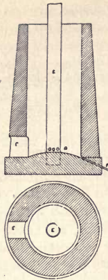
FIG. 172—The Hahnemann Peat Coking Oven.
