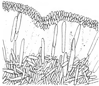
Fig. 17. Querschnitt durch die Stielrinde von Cavernularia chuni . Vergr. 25.
