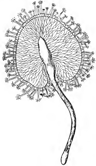
Fig. 32. Renilla amethystina , Ventralfläche.
