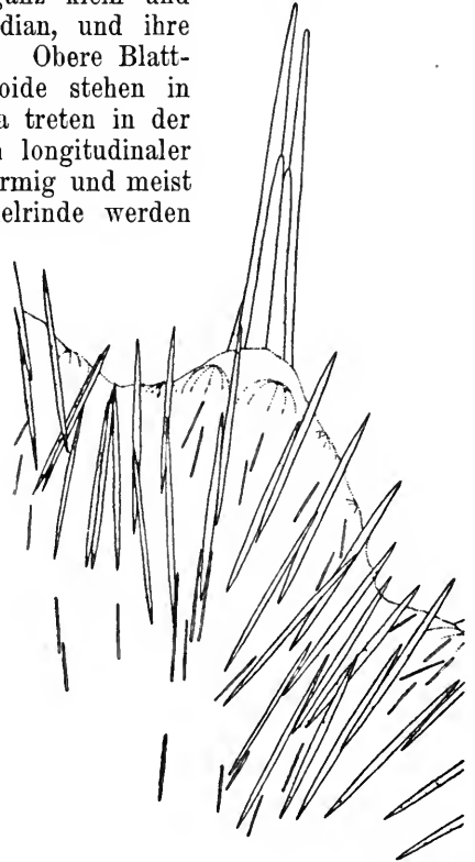
Fig. 108. Polypenzone der Blattoberseite von Pteroeides lusitanicum . Vergr. 13.
