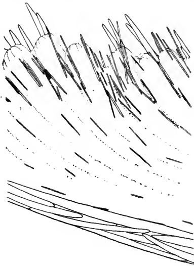
Fig. 112. Polypenzone der Blattoberseite von Pteroeides sagamiense . Vergr. 13.
