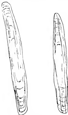
Fig. 28. Kielspicula von Renilla edwardsii . Vergr. 100.
