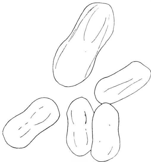
Fig. 23. Spicula der Stielrinde von Actinoptilum molle . Vergr. 100.
