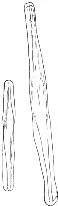
Fig. 30. Spicula der Stielrinde von Renilla mülleri . Vergr. 100.
