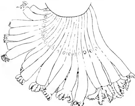
Fig. 73. Unterseite eines Blattes von Virgularia schultzei . Vergr. 14.
