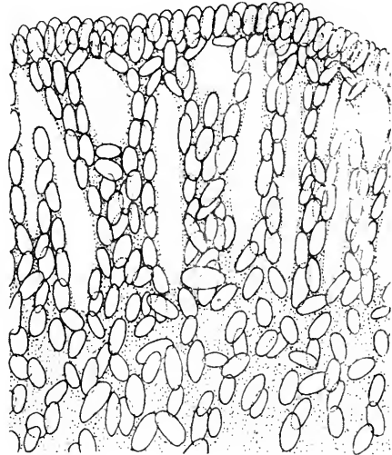
Fig. 14. Querschnitt durch die Stielwand von Cavernularia obesa . Vergr. 25.
