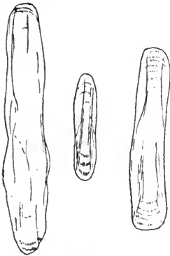
Fig. 33. Spicula der Stielrinde von Renilla amethystina . Vergr. 100.
