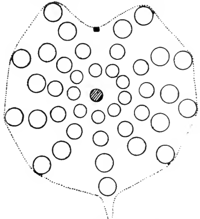
Fig. 57. Diagramm des Polypenstandes von Umbellula antarctica.
