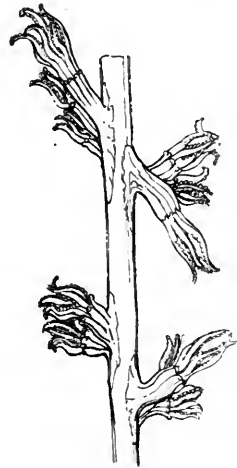
Fig. 75. Ein Stück der Kolonie von Virgularia tuberculata. Stärker vergrößert. (Nach A. M. Marshall.)
