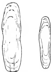
Fig. 27. Spicula der Stielrinde von Renilla edwardsii . Vergr. 100.
