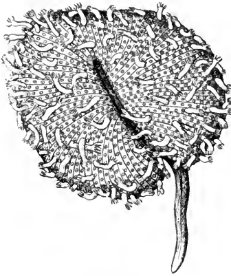
Fig. 31. Renilla amethystina , Dorsalfäche.
