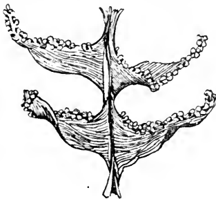
Fig. 65. Ein Stück des Polypars von Scytalium martensii . (Nach Thomson & Henderson.)
