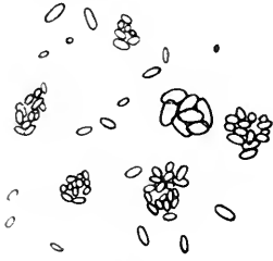
Fig. 76. Spicula des Stielinneren von Virgularia mirabilis . Vergr. 370.
