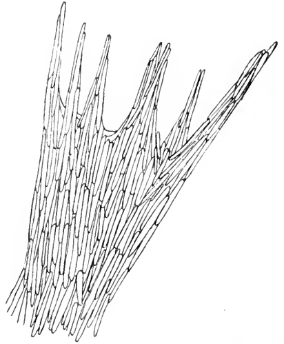
Fig. 82. Spicula des Polypenkelches von Pennatula inflata .
