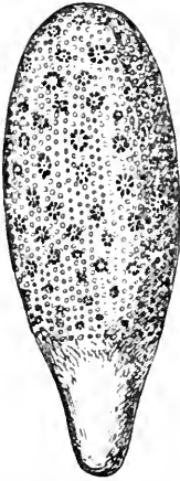
Fig. 15. Cavernularia lütkenii . (Nach Kölliker.)
