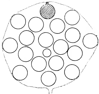
Fig. 59. Diagramm des Polypenstandes von Umbellula pellucida .
