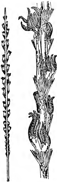
Fig. 68. Stylatula elegans. (Nach A. M. Marshall.) Rechts ein Stück der Kolonie vergrößert.
