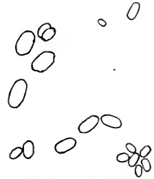
Fig. 77. Spicula des Stielinneren von Virgularia gustaviana . Vergr. 370.
