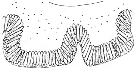
Fig. 18. Querschnitt durch die Stielrinde von Cavernularia clavata . Vergr. 25.
