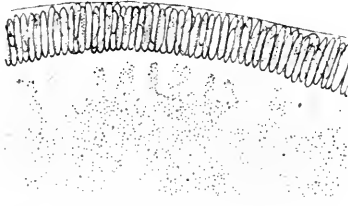
Fig. 19. Querschnitt durch die Stielrinde von Cavernularia pusilla . Vergr. 25.
