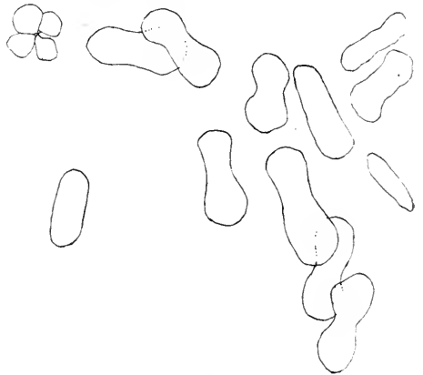
Fig. 13. Spicula vom Stiel und unteren Teil des Polypars von Veretillum cynomorium .
