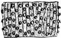
Fig. 22. Actinoptilum molle . Ein Stück der Kieloberfläche.
