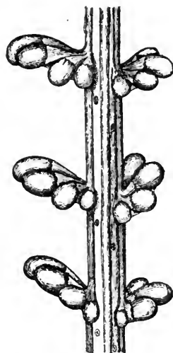
Fig. 67. Scyталиopsis djiboutiensis . Ein Stück des Polypars vergrößert. (Nach Gravier.)
