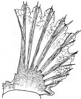
Fig. 120. Blatt aus der Mitte der Feder von Struthiopterion caledonicum. Vergr. 3.
