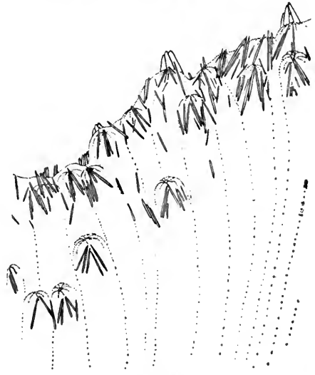
Fig. 113. Polypenzone der Blattoberseite von Pteroeides jungerseni . Vergr. 13.
