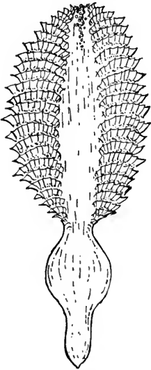
Fig. 104. Pteroeides griseum . (Nach Niedermeyer.)
