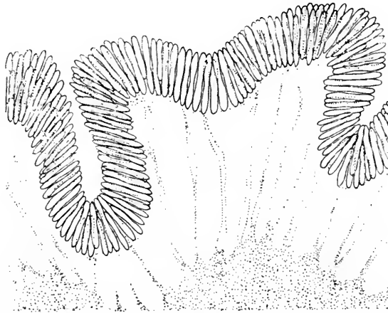
Fig. 20. Querschnitt durch die Stielrinde von Cavernularia elegans . Vergr. 25.
