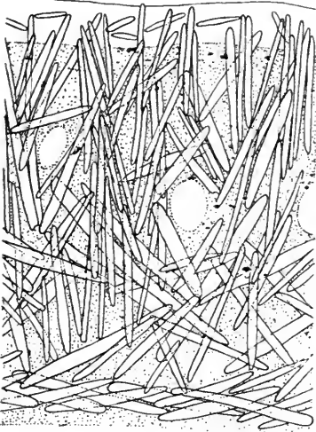
Fig. 16. Querschnitt durch die Stielrinde von Cavernularia glans . Vergr. 25.
