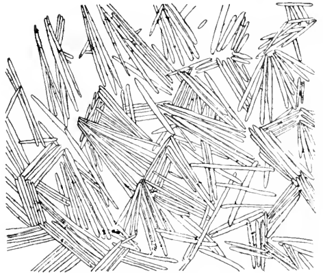
Fig. 83. Spicula der dorsalen Kielzooide von Pennatula inflata .
