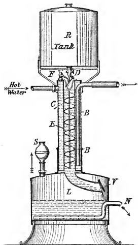
FIG. 314.— SIMPLEX CARBURETTOR.
