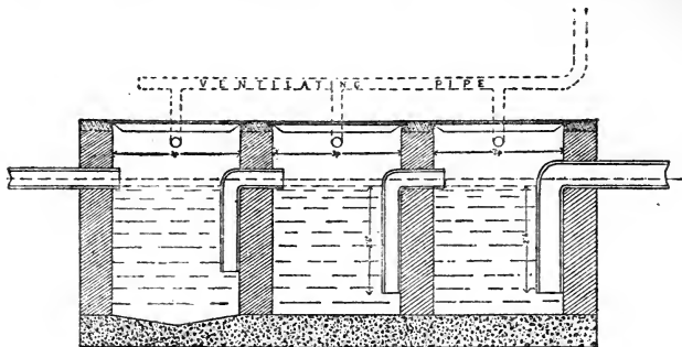
Longitudinal Section.
