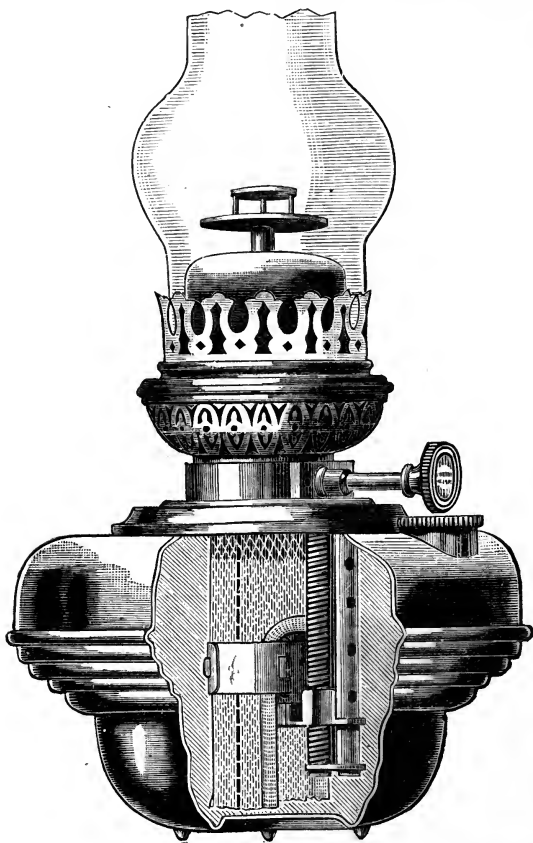
FIG. 296.—LAMPE VERITAS.
