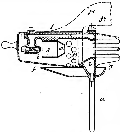
FIG. 307.—WELLS LAMP.
