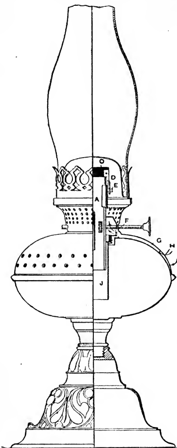
FIG. 301.—VICTORIA LAMP.
