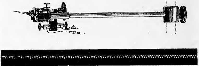
Fig. 5. — Appareil à signaux électriques de M. Deprez; signaux de cet appareil actionné par un diapason interrupteur de 500 vibrations simples par seconde. (Héliogravure.)
