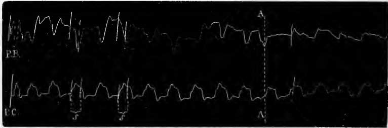
Fig. 120. — PB, variations de la pression buccale exprimant les changements de volume du cœur.—PC, pulsations du cœur.—S, systoles. Pulsations des artères bucco-pharyngiennes quand la glotte est fermée, à partir de AA.
