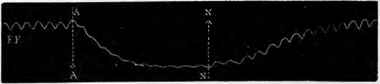
Fig. 62. — Comparaison des effets produits par la compression des veines caves en AA' sur la pression fémorale (PF) et des résultats de la contre-pression exercée sur le cœur. En NN', on rétablit le cours du sang veineux.
