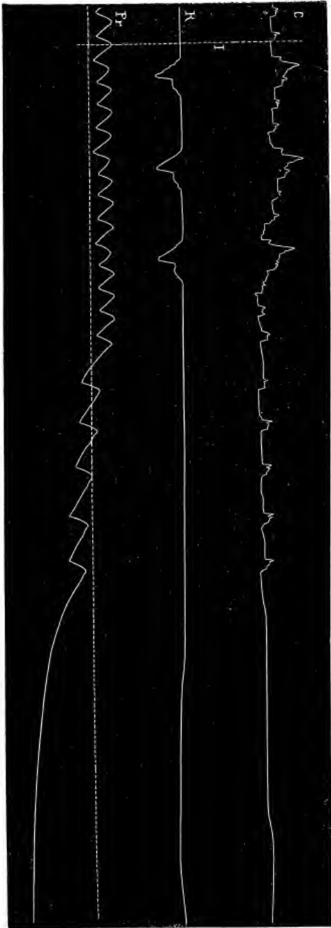
Fig. 82. — Effets immédiats de l'injection de chloral faite dans la veine jugulaire d'un chien de 13 kilogr. (4 gramme de chloral dans 3 centim. cubes d'eau). — I, instant de l'injection. — C, pulsations du cœur avec courbes respiratoires. — R, courbes de la respiration recueillies avec le pneumographe. — Pr, pression artérielle.
