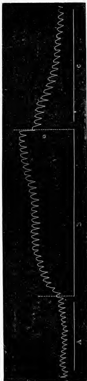
Fig. 8. — Turgescence du cerveau Ce, quand la malade incline la tête et le tronc en avant le E en E'.
