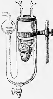
Fig. 95. — Appareil à déplacement pour l'étude des changements de volume du cœur isolé : V, tube d'afflux ; — A, tube d'écoulement artériel.
