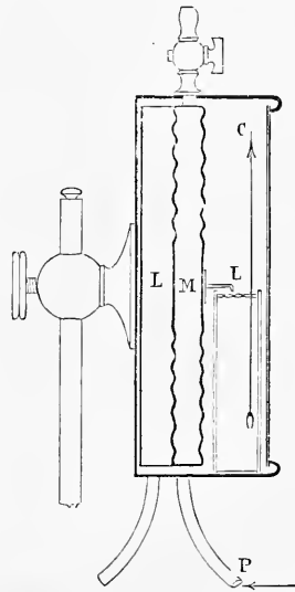
Fig. 150. — Manomètre à cadran et à transmission.
