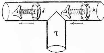
Fig. 155. — Tube à double soupape se montant sur la canule trachéale à la place du pavillon montré en place dans la figure précédente.
