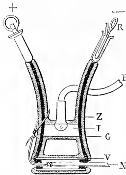
Fig. 457. Excitateur isolé. — P, tige en plomb fixée à une plaque d'ivoire I ; Z, tige de zinc amalgamé formant conducteur ; V, tube de verre isolant les deux zincs ; G, gutta-percha isolant l'appareil ; N, nerf introduit dans le tube excitateur et fixé avec un fil. (Le fil doit toujours être introduit par le plus petit orifice avant la ligature du nerf : c'est par le glissement de ce fil dans l'anneau qu'on attire le nerf dans le tube).
