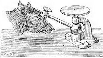
Fig. 459. Appareil contentif pour le rat. Le même modèle sert à fixer la tête du chat.
