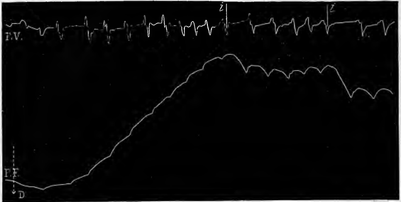
Fig. 67. — Phénomènes artériels et cardiaques qui suivent la décompression du cœur, faite en D. On voit la pression fémorale (PF) se relever très-rapidement et les pulsations du cœur (PV) présenter les caractères des pulsations à forte réplétion diastolique. En ii , deux intermittences.
