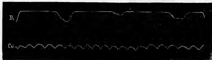
Fig. 71. — R, courbes des respirations thoraciques recueillies avec le pneumographe. Ce, Mouvements du cerveau; ils ne présentent plus les oscillations respiratoires que l'on constate dans la figure précédente.
