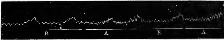
Fig. 42. — Pulsations du cœur d'un lapin profondément chloralisé. — Phases d'accélération AA. — Ralentissement des pulsations pendant les phases RR.
