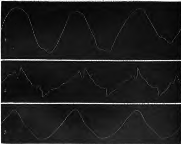
Fig. 34. — Courbes des mouvements d'élévation et d'abaissement de l'aile. 1. Courbe recueillie sur le pigeon par M. Marey. 2. Courbe d'un oiseau mécanique à ressort de caoutchouc. 3. Courbes des mouvements de l'aile de l'appareil mécanique à air comprimé. On remarque l'analogie de cette dernière avec celle obtenue sur la nature.
