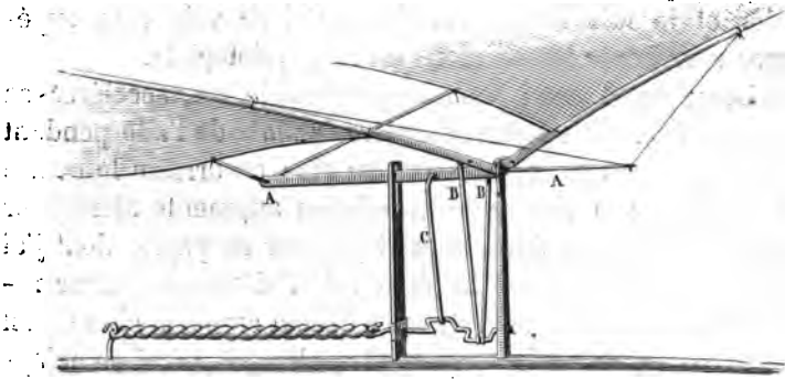
Fig. 35. — AA. Axe commun des ailes. — BB. Bielles produisant l'élévation et l'abaissement des ailes. C. Bielle produisant l'inclinaison de l'axe des ailes, ce qui donne le changement de plan.
