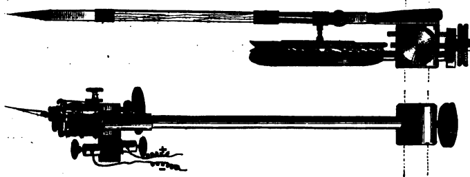
Fig. 65. — Disposition pour l'inscription simultanée du mouvement des lèvres et des vibrations du larynx.
