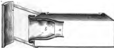
Fig. 154. — Coupe de l'appareil destiné à comprimer la main et l'avant-bras, a . — Manchon de caoutchouc invaginé dans la caisse, b . — Manchon de taffetas supprimant l'extensibilité du 1 er manchon. Une pièce retenue par des courroies empêche le bras de céder à la pression intérieure.
