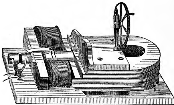
Saxton-Ettinghausen Apparatus.
