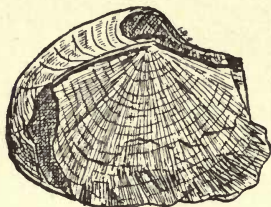
FIG. 19.— Productus . Coal-measures.
