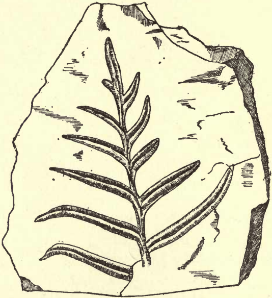
FIG. 5.— Pecopteris Serlii . Coal-shale.
