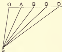
FIG. 59.
