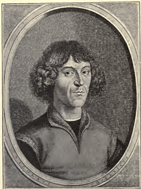
FIG. 3.—Copernicus.
