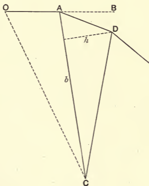
FIG. 70.
