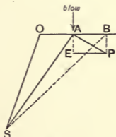
FIG. 61.
