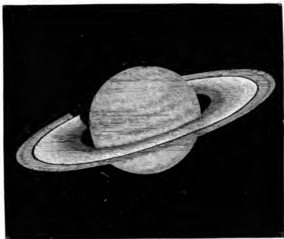
FIG. 81.—Saturn.
