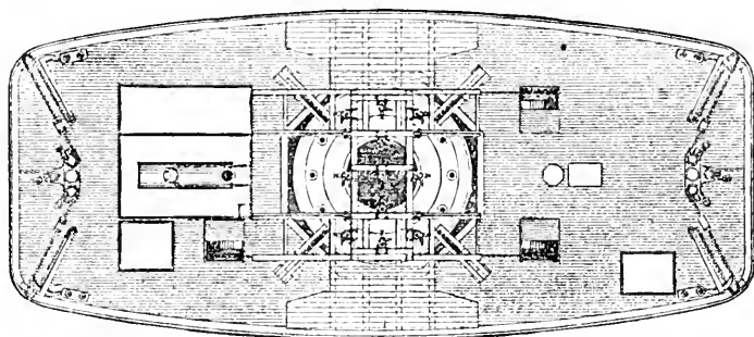
FIG. 2.—DECK PLAN.
