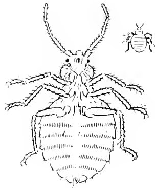
FIG. 17. ACANTHIA INODORA
