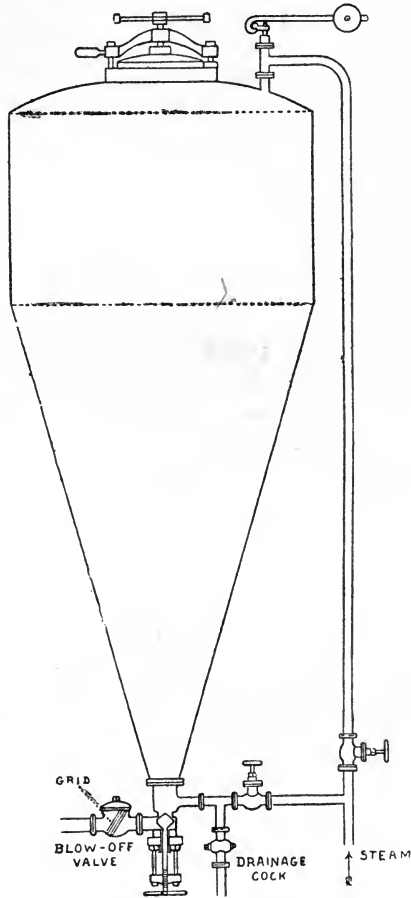
FIG. 3.—Henze Convertor.
