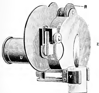
FIG. 92.—DARE'S HEMOGLOBINOMETER. (Da Costa.)
