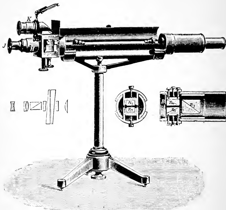
FIG. 7.—POLARISCOPE (SCHMIDT AND HÄNSCH MODEL).
