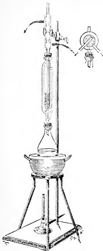
FIG. 108.—SOXHLET APPARATUS.
