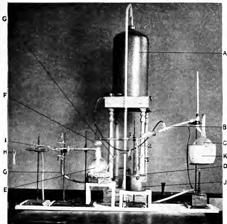
FIG. 24.—FISCHER APPARATUS.
