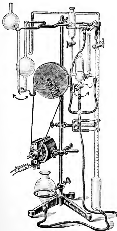
FIG. 34.—VAN SLYKE AMINO NITROGEN APPARATUS.
