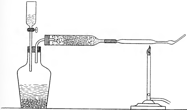
FIG. 131.—MARSH APPARATUS.
