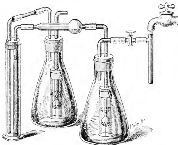
FIG. 163.—FOLIN AMMONIA APPARATUS.
