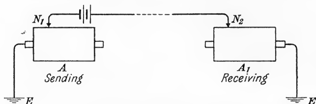
FIG. 10.—Bakewell's Apparatus.
