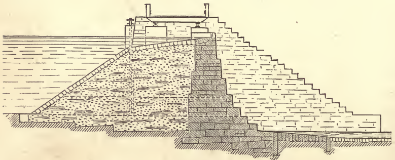
WASTE-WEIR.
