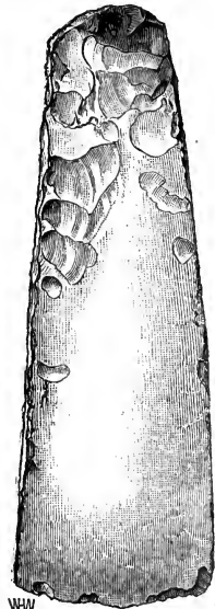
Stone Axe.
