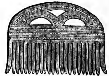
Comb.
