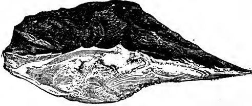
Awl.
