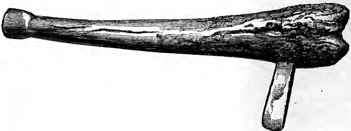
African Axe.
