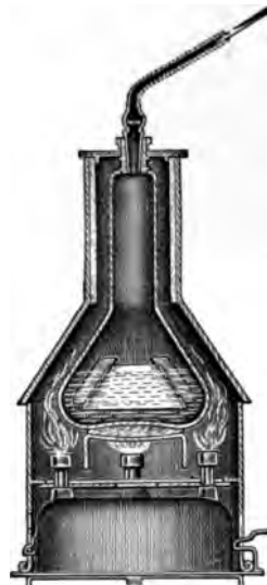
FIG. 62.—Formaldehyd gas regenerator.
