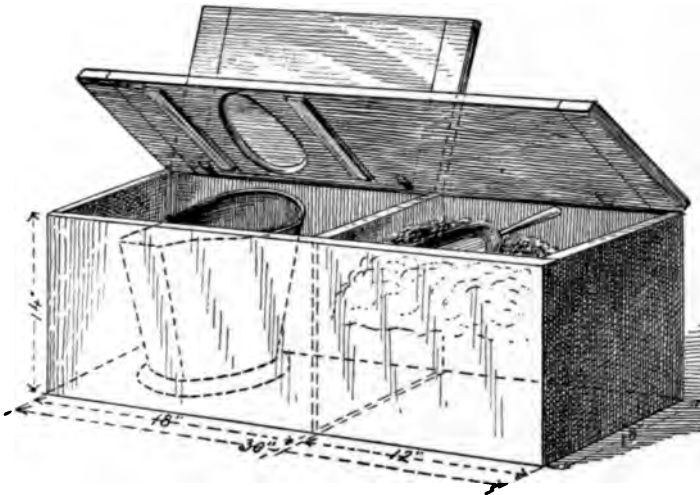
FIG. 42.—Dry-earth closet.
