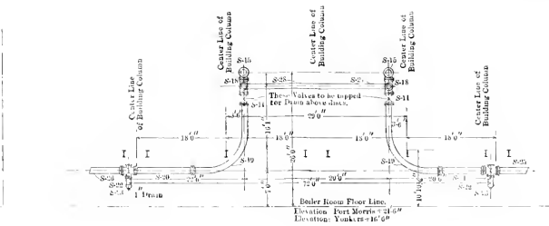
ELEVATION A-A
