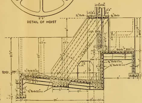
LONGITUDINAL SECTION J-I
