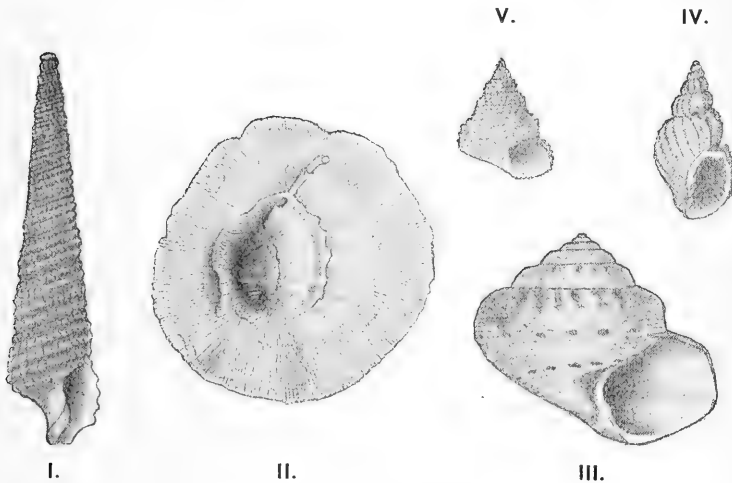
FIG. I. Terebra Walkeri , n.sp. \times 2 . ,, II. Coralliochia fimbriata , A. Ad. \times 2 . ,, III. Monilia simulans , n.sp. \times 2 . ,, IV. Cancellaria pallida , n.sp. \times 2 . ,, V. Calliostoma deceptum , n.sp. \times 2 .
