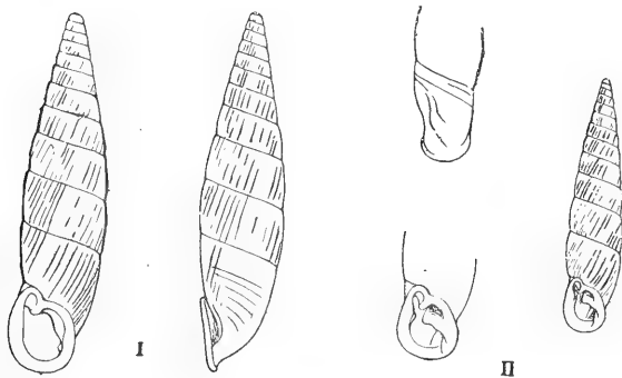
FIG. I. Clausilia timalthea , n.sp.
