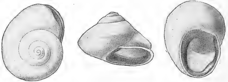
FIG. VI. Papuina chilochoa , n.sp.
