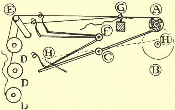
FIG. 17. DOUBLER
