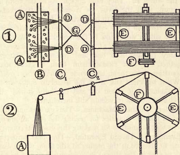
FIG. 13. REELING MACHINE
