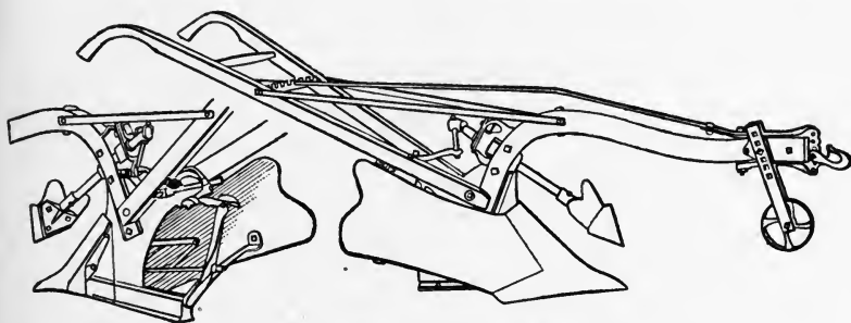
FIG. 84.—Hillside plow. (Walking type.)
