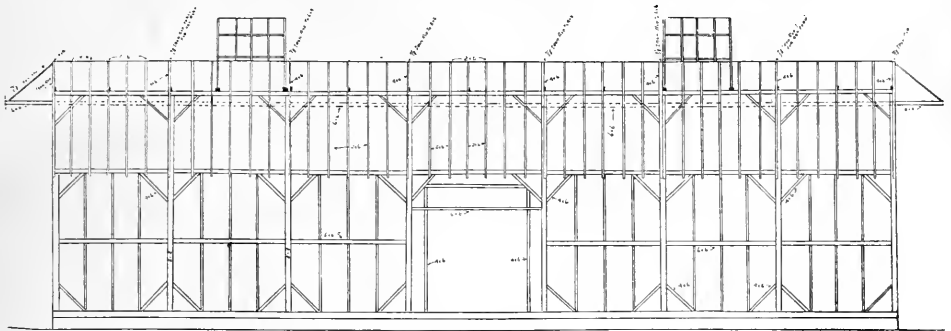
LONGITUDINAL SECTION
