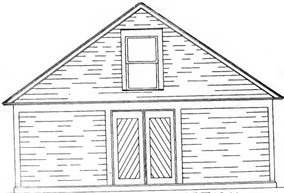
END ELEVATION
