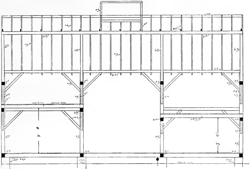
LONGITUDINAL SECTION
