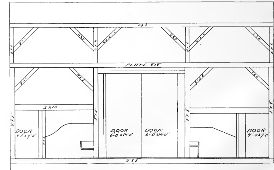
LONGITUDINAL SECTION
