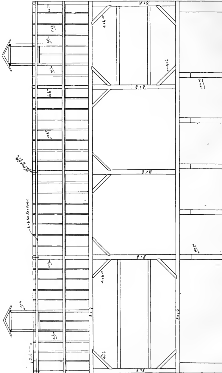
LONGITUDINAL SECTION
