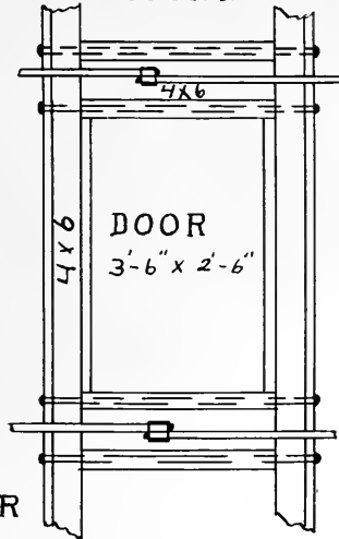
DOOR SECTION
