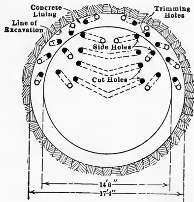
FIG. 22.—Heading Holes.
