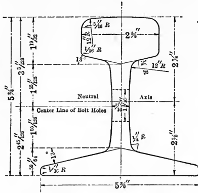
FIG. 70.—A. S. C. E. 90-lb. Rail.
