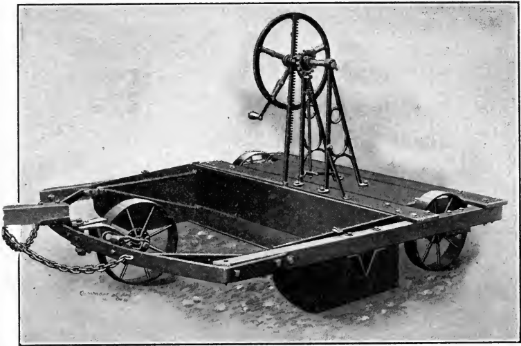
FIG. 3.—Shuart Grader.
