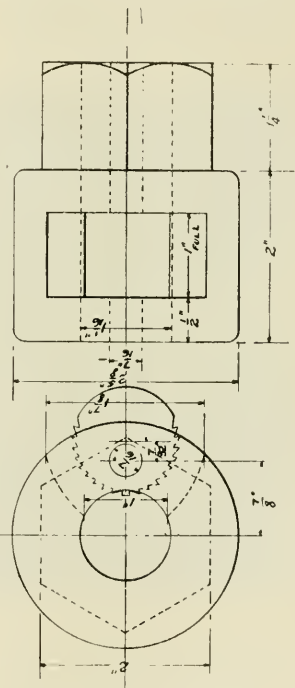
FIG. 2—STUD WRENCH.
