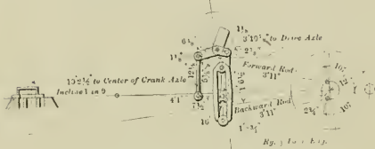
FIG. 29. ALLAN STRAIGHT LINK.
