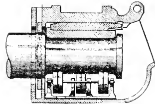
JOURNAL LUBRICATOR.
