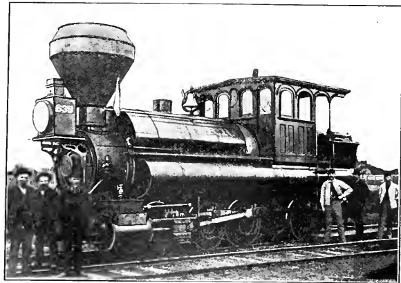
FIG. 2. OLD WOOD-BURNING TANK ENGINE, NO. 685, J. M. & I. R. R.
