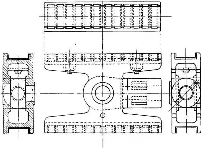
CORED STEEL CROSSHEAD, L. & N. E.
