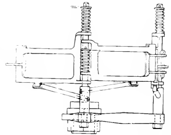
FIG. 1—LUBRICATOR GUARD FRAME
