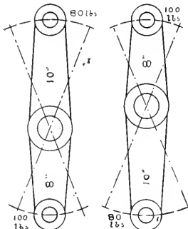
FIG. 1. ROCKER ARMS
