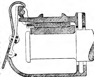
JOURNAL BOX LID.
