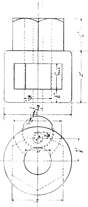
FIG. 2—STUD WRENCH.
