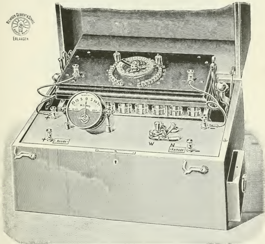
Transportable Chromsäure-Tauchbatterie.
