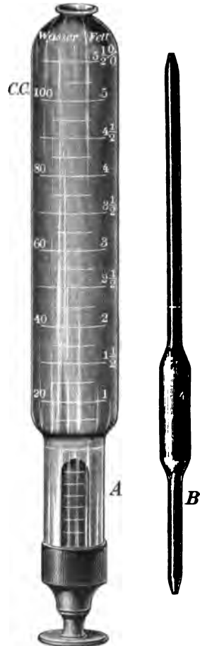
FESERs Laktoskop.
