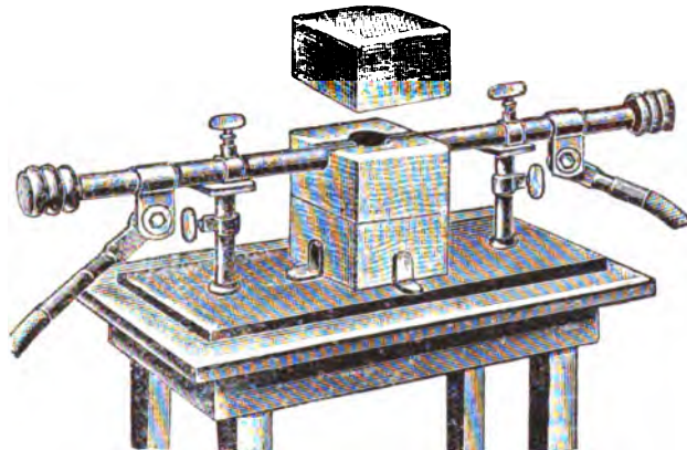
Versuchsöfen mit Heizung durch den elektrischen Flammenbogen.
