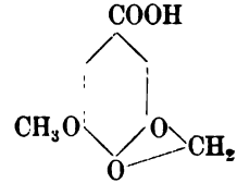
Myristicinsäure
