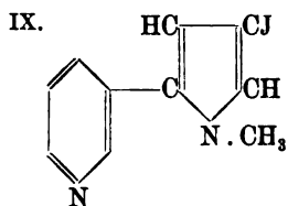
Jodnicotyrin.
