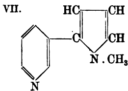
N-β-Pyridylpyrrol.
