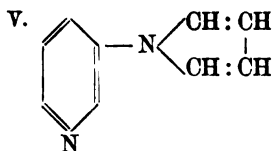
N-β-Pyridylpyrrol.
