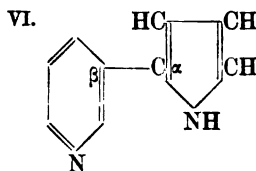
C-αβ-Pyridylpyrrol.
