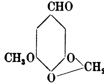
Myristinaldehyd
