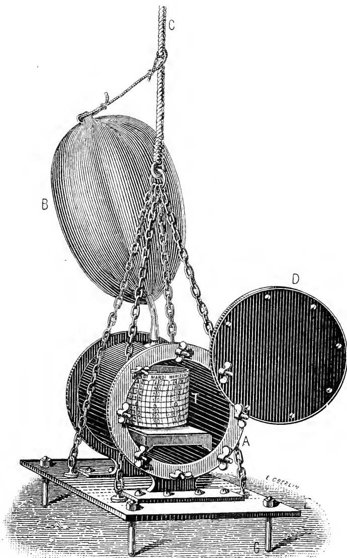
Fig. 147. — Thermomètre enregistreur de P. Regnard pour obtenir en courbe continue la température du fond des mers.
