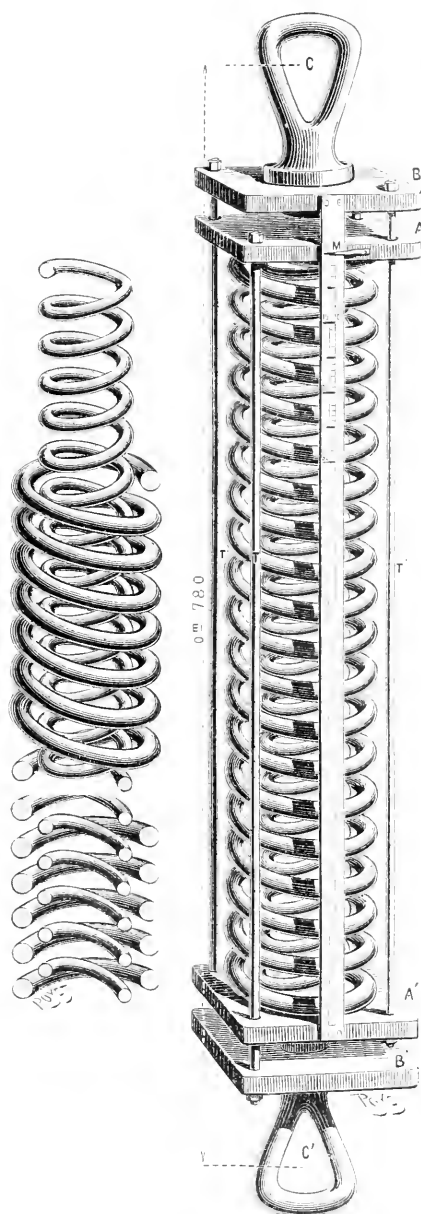
Fig. 9. — Accumulateur de l'Hirondelle.
