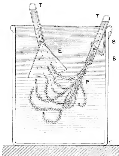
Fig. 123. — Appareil de Devaux pour l'étude de l'atmosphère superficielle et de l'atmosphère interne des plantes submergées.
