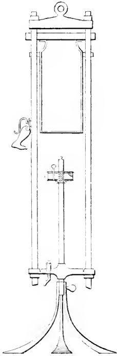
Fig. 167. — Bouteille d'Elkmann.
