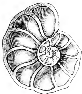
Fig. 26. — Nanionina crassula .
