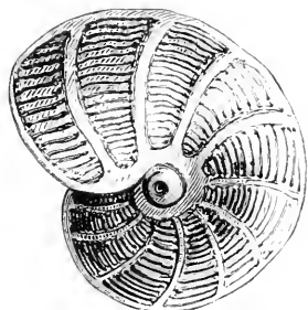
Fig. 28. — Peneroplis planatus .
