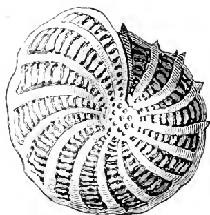
Fig. 27. — Polystomella crispa .
