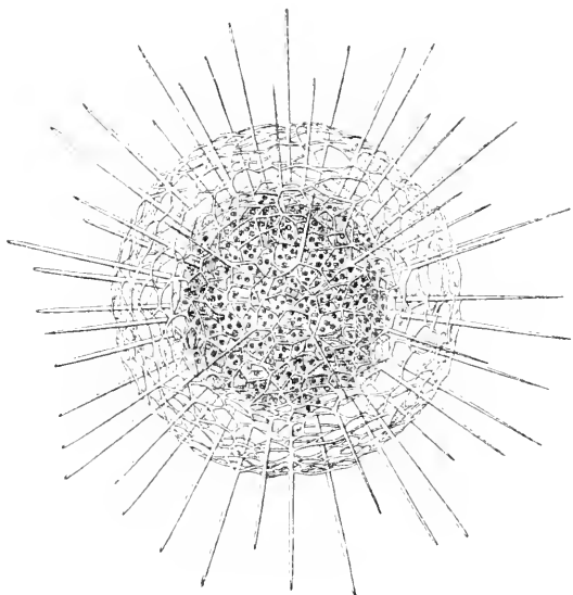
Fig. 32. — Haliomma .
