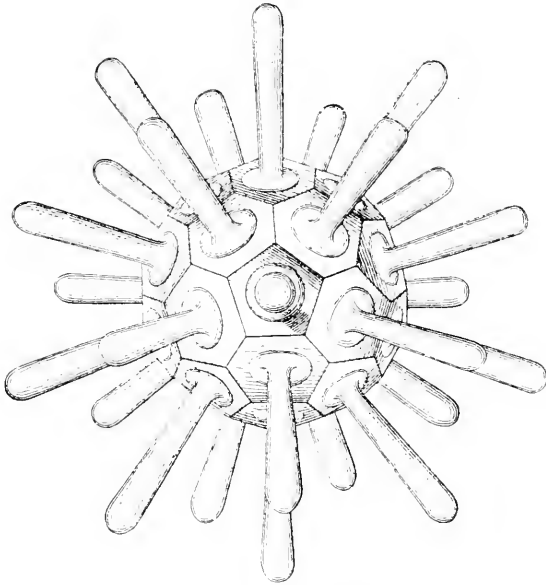
Fig. 37. — Rhabdosphère .
