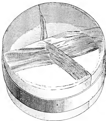
Fig. 87. — Hublot de quartz brisé à l'essai par une pression de 450 atmosphères.
