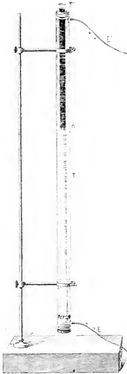
Fig. 177. — Dispositif destiné à mesurer la rapidité de la diffusion de l'oxygène dans l'eau.
