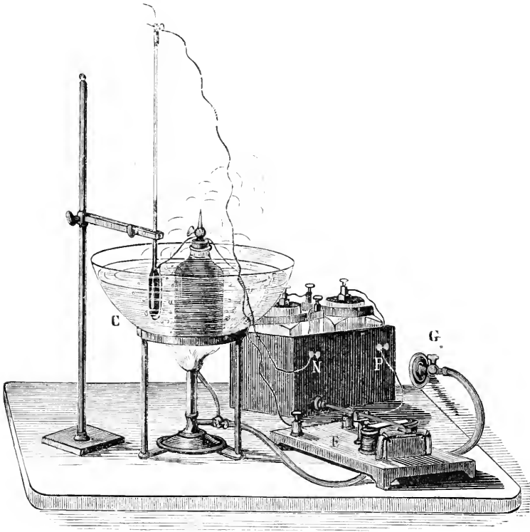
Fig. 78. — Thermostat électrique.
