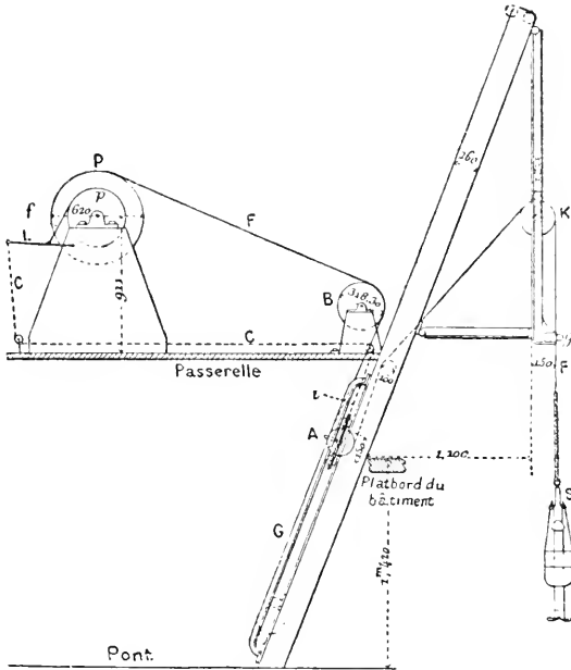
Fig. 63. — Machine à sonder du Talisman .
