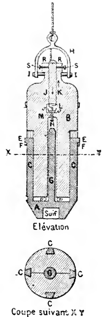
Fig. 58. — Sonde électrique de Delacroix.
