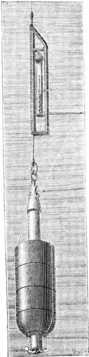
Fig. 57. — Sonde du Talisman .
