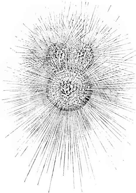
Fig. 21. — Globigerina bulloides .
