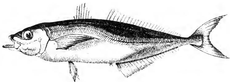
Fig. 206. — Caranx Trachurus .
