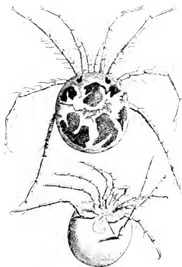
Fig. 48. — Campognatha Forelli .
