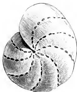
Fig. 29. — Polystomella umbiliculata .
