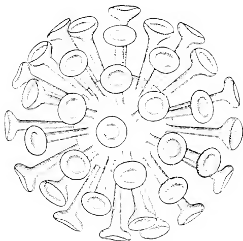
Fig. 36. — Rhabdosphere .
