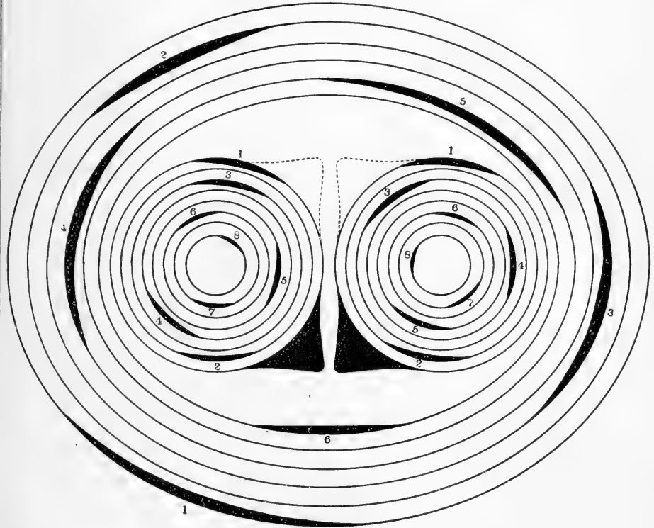
Fig. 3. Diagramm des zweiten Verästelungsstückes. Die Längen der sechs Knospen des Fussesstückes sind den beobachteten Längen dieser Knospen proportional gezeichnet.
