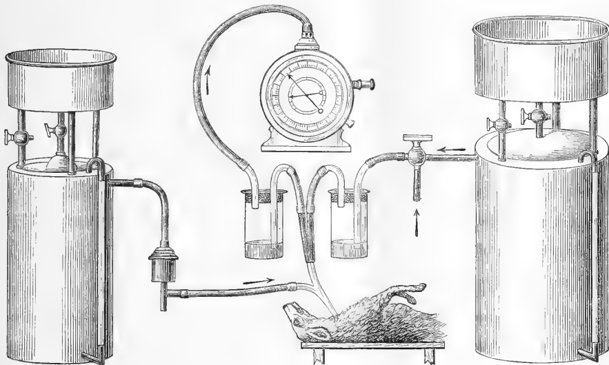
APPARECCHIO PER LA RESPIRAZIONE DEL GAS ACETILENE.
