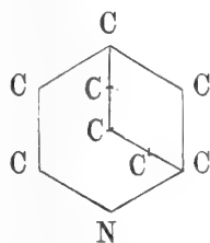
Schema delle basi granataniche
