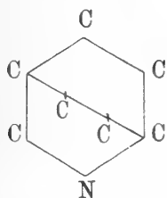
Schema delle basi tropiniche
