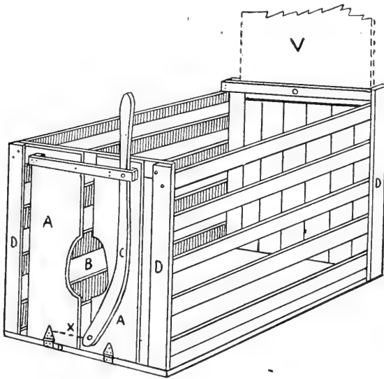
Fig. 317. Hog Trap.
