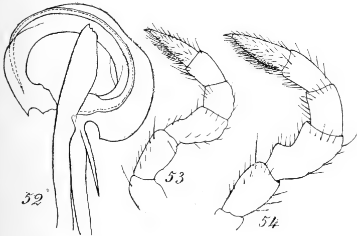
FIG. 52. Distale Hälfte eines Gonopodentelopodits. — FIG. 53. Bein des 1. Paares. — FIG. 54. Bein des 2. Paares.
