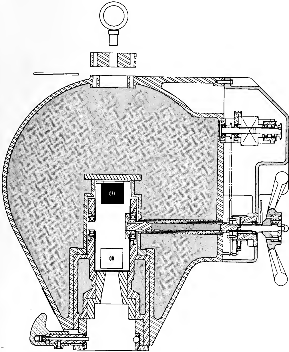
Fig. 1—Keleket-Barnes source shield.
