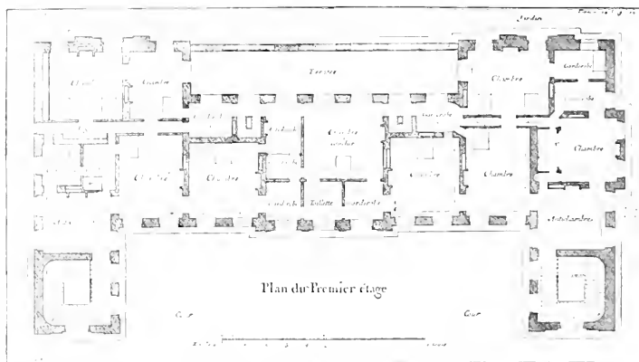
Grundriß zum Landhaus eines adligen Herrn. Aus Blondel: De la distribution des maisons de plaisance. Paris 1737.
