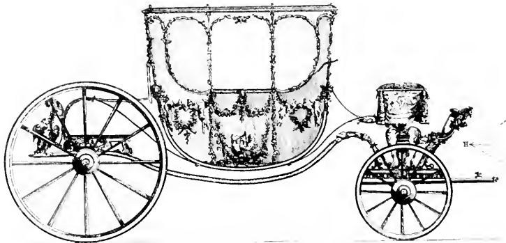
Entwurf zu einer Berline. Zeichnung von Mercier. 1776
